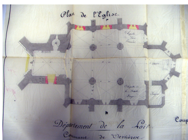
Département de la Loire. Commune de Verrières. Plans, coupe et élévation de l'église de cette commune [..]. Plan de l'église. Encre, plume et lavis coloré sur calque, échelle 0,002 m pour 1 m, 57,5x66,5. 16 mai 1846 AD Loire. V 917 Repro. Caroline Guibaud, Autr. Dulac (agent voyer) IVR82_20104200272NUCA
