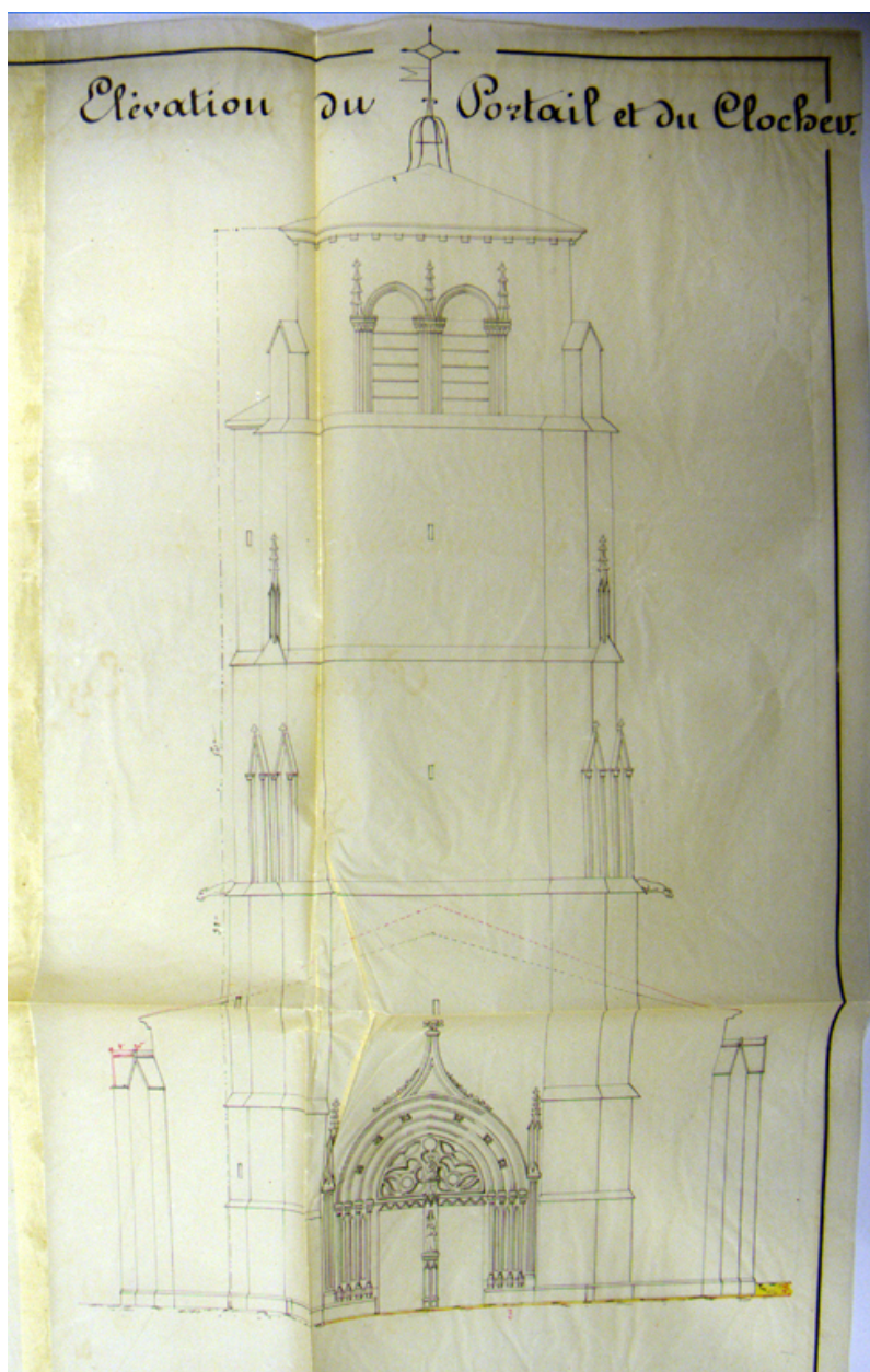
Département de la Loire. Commune de Verrières. Plans, coupe et élévation de l'église de cette commune [...]. Elévation du portail et du clocher. Encre, plume et lavis coloré sur calque, échelle 0,002 m pour 1 m, 57,5x66,5. 16 mai 1846 AD Loire. V 917
