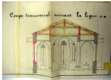
Département de la Loire. Commune de Verrières. Plans, coupe et élévation de l'église de cette commune [...]. Coupe transversale suivant la ligne AB. Encre, plume et lavis coloré sur calque, échelle 0,002 m pour 1 m, 57,5x66,5. 16 mai 1846 AD Loire. V 917 Repro. Caroline Guibaud, Autr. Dulac (agent voyer) IVR82_20104200274NUCA
