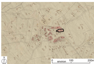
Plan de situation, d'après le cadastre de 1810 (?), section D, échelle originale 1:2500. Plan cadastral, dit cadastre napoléonien. Dessin au crayon, plume et lavis d'encre colorées sur papier, 1810. AD Loire. 3P-1682VT Dess. Caroline Guibaud IVR82_20104200279NUD
