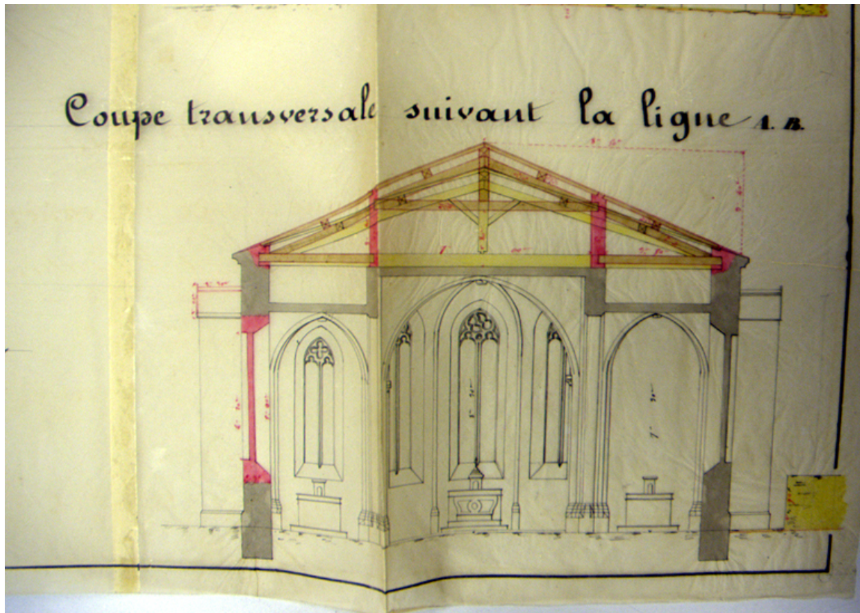
Département de la Loire. Commune de Verrières. Plans, coupe et élévation de l'église de cette commune [...]. Coupe transversale suivant la ligne AB. Encre, plume et lavis coloré sur calque, échelle 0,002 m pour 1 m, 57,5x66,5. 16 mai 1846 AD Loire. V 917
