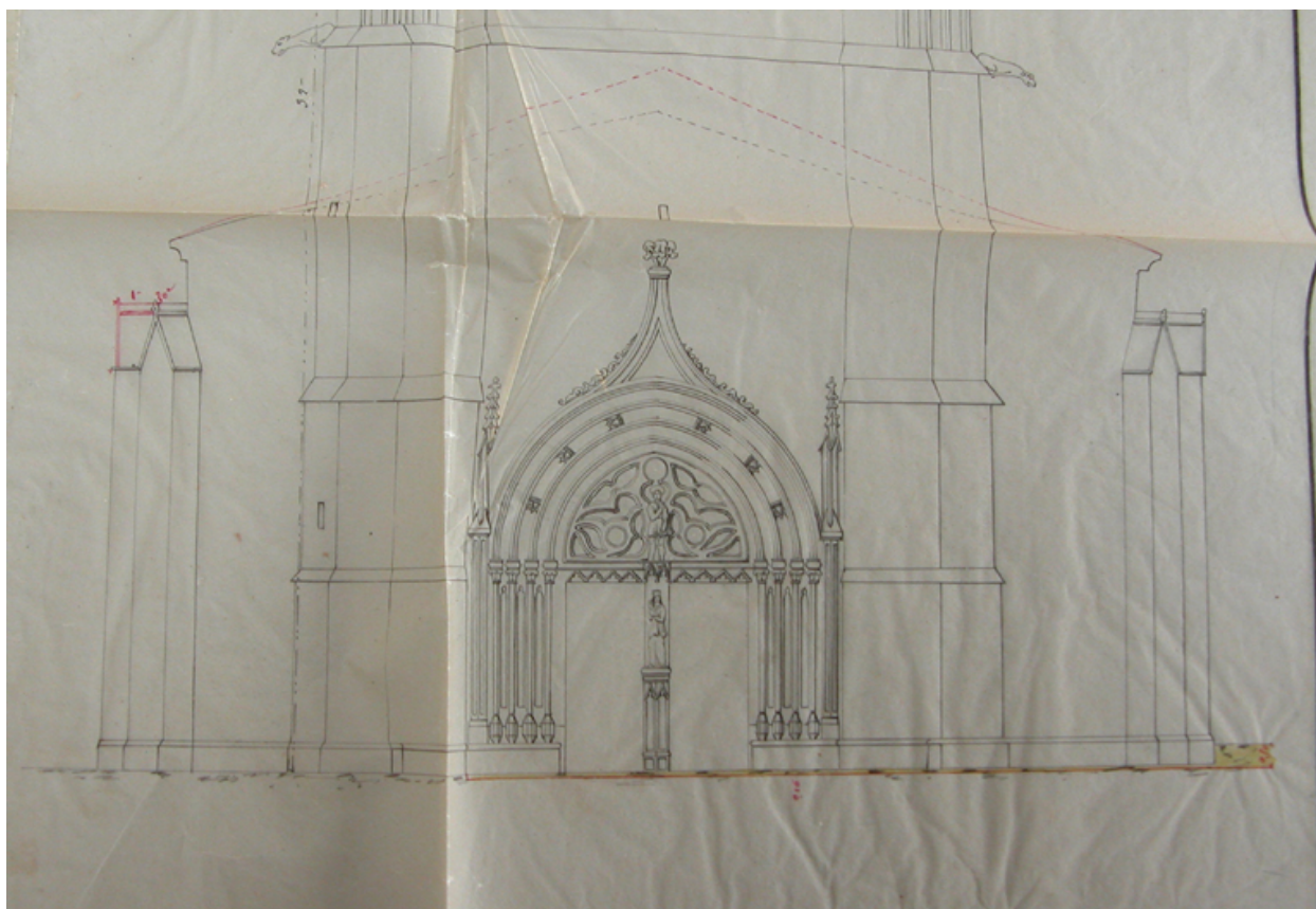
Département de la Loire. Commune de Verrières. Plans, coupe et élévation de l'église de cette commune [...]. Elévation du portail et du clocher. [Détail du portail]. Encre, plume et lavis coloré sur calque, échelle 0,002 m pour 1 m, 57,5x66,5. 16 mai 184
