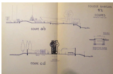
Plan coupe (Grimal, 1976) (AN 19880466/114). Autr. Franck Grimal, Repro. Valérie Pamart IVR84_20206900370NUCA
