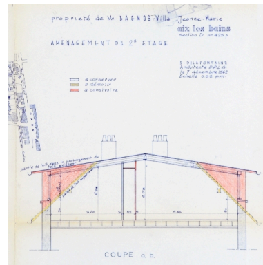
Aménagement de l'étage de combles : coupe Repro. François Fouger IVR82_20117300261NUCB
