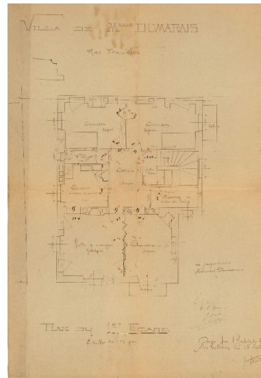
Plan du 1er étage Repro. François Fouger IVR82_20117300258NUCB
