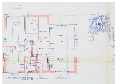
Aménagement de l'étage de combles : plan Repro. François Fouger IVR82_20117300260NUCB
