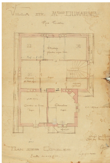
Plan des combles Repro. François Fouger IVR82_20117300259NUCB
