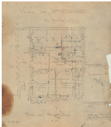
Plan du sous-sol Repro. François Fouger IVR82_20117300256NUCB
