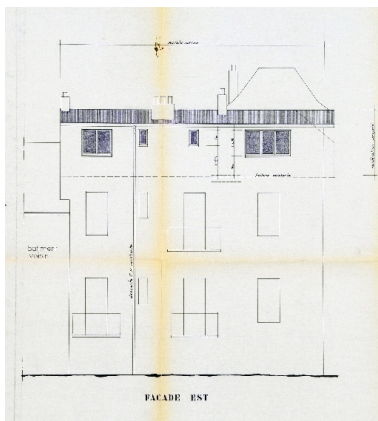
Aménagement de l'étage de combles : élévation est Repro. François Fouger IVR82_20117300263NUCB
