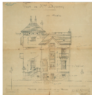
Elévation occidentale Repro. François Fouger IVR82_20117300254NUCB
