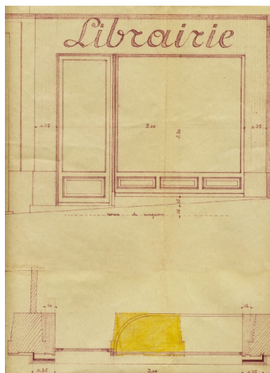
Projet de transformation de la façade Repr. François Fouger, Autr. Bellet et Pinson IVR82_20037300024NUCB
