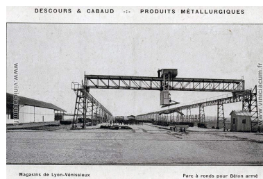
Descours et Cabaud - Produits métallurgiques - Magasins de Lyon-Vénissieux - Parc à ronds pour béton armé (Association Viniciacum) Phot. Alice Giacovelli IVR84_20226900410NUC
