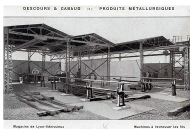
Descours et Cabaud - Produits métallurgiques - Magasins de Lyon-Vénissieux - Machine à redresser les fils (Association Viniciacum) Phot. Alice Giacovelli IVR84_20226900406NUC
