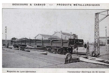
Descours et Cabaud - Produits métallurgiques - Magasins de Lyon-Vénissieux - Transbordeur électrique de 60 tonnes (Association Viniciacum) Phot. Alice Giacovelli IVR84_20226900405NUC
