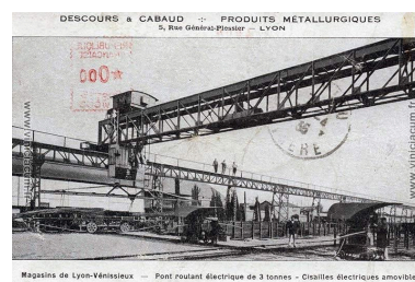
Descours et Cabaud - Produits métallurgiques - Magasins de Lyon-Vénissieux - Pont roulant et cisailles électriques (Association Viniciacum) Phot. Alice Giacovelli IVR84_20226900407NUC
