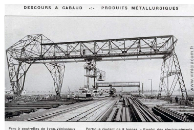
Descours et Cabaud - Produits métallurgiques - Magasins de Lyon-Vénissieux - Portique roulant (Association Viniciacum) Phot. Alice Giacovelli IVR84_20226900413NUC
