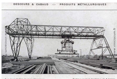
Descours et Cabaud - Produits métallurgiques - Magasins de Lyon-Vénissieux - Portique roulant électrique (Association Viniciacum) Phot. Alice Giacovelli IVR84_20226900412NUC
