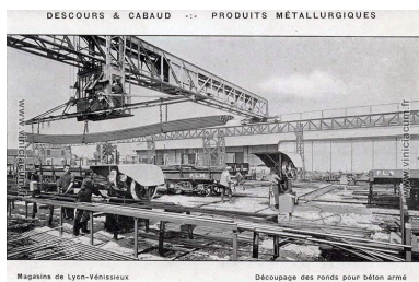
Descours et Cabaud - Produits métallurgiques - Magasins de Lyon-Vénissieux - Découpage des ronds pour béton armé (Association Viniciacum) Phot. Alice Giacovelli IVR84_20226900408NUC
