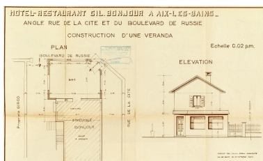
plan et élévation de la véranda Repro. François Fouger IVR82_20057300869NUCB
