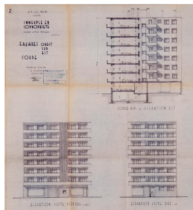
Immeuble Le Régent et garage de réparation automobile. Élévations et coupe, 1957 Repr. Denys Harreau IVR84_20167300065NUCB
