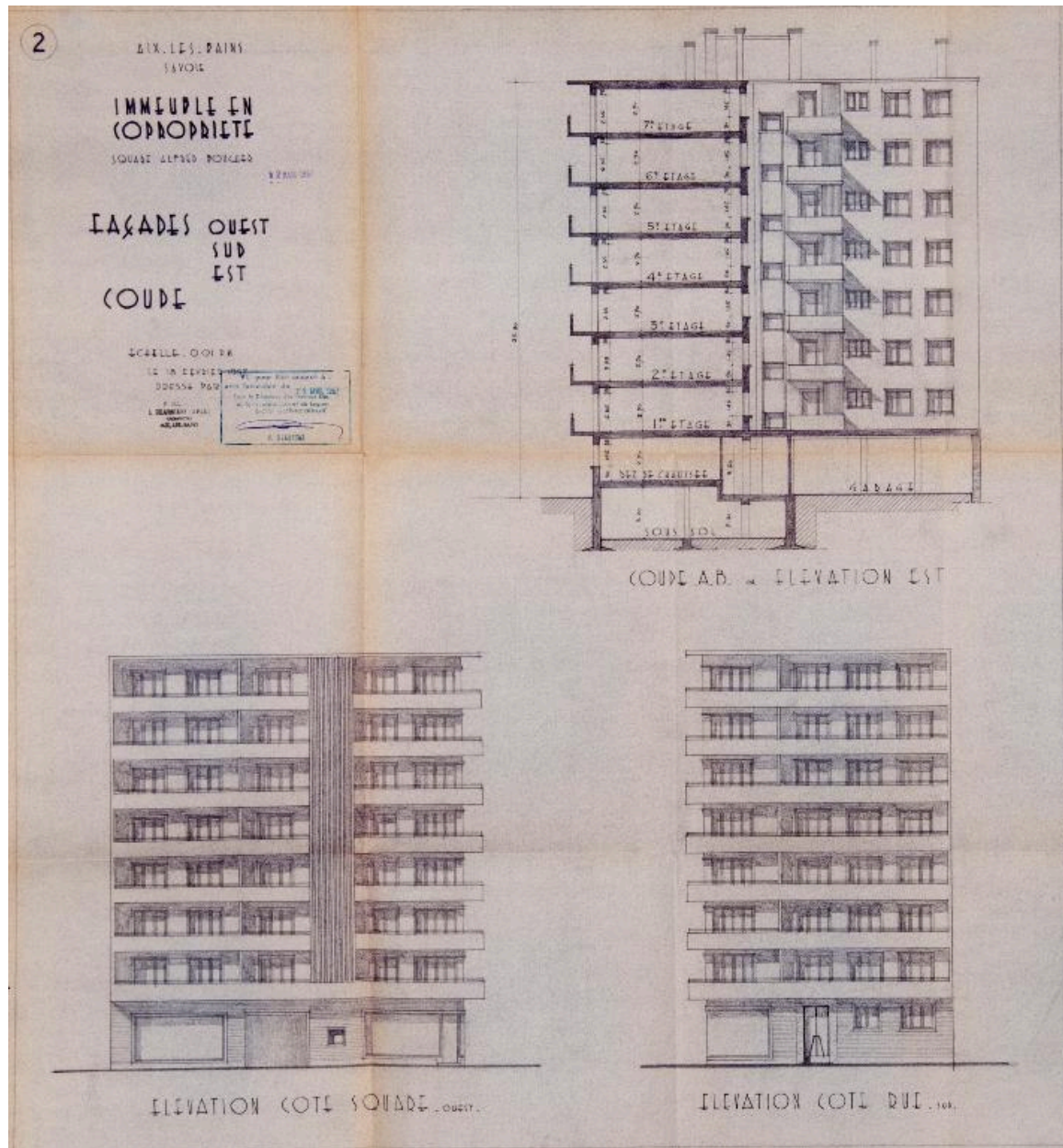
Immeuble Le Régent et garage de réparation automobile. Élévations et coupe, 1957
