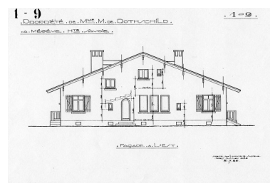
Elévation orientale / Henri Jacques Le Même, 31 juillet 1926 Phot. F. Véry, Autr. Le Même Henry Jacques (architecte) IVR82_20127402168NUC
