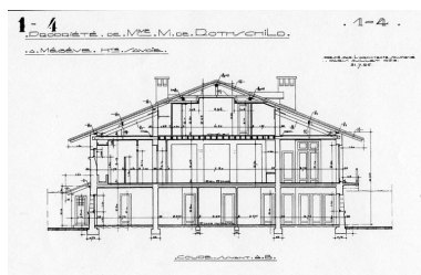
Coupe longitudinale / Henri Jacques Le Même, 31 juillet 1926 Phot. F. Véry, Autr. Le Même Henry Jacques (architecte) IVR82_20127402164NUC
