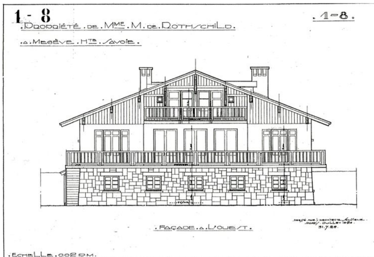
Elévation ouest. Henry Jacques Le Môme, 31 juillet 1926
