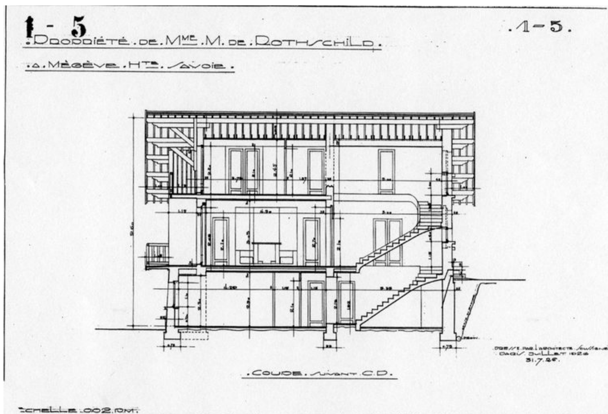
Coupe transversale / Henri Jacques Le Même, 31 juillet 1926
