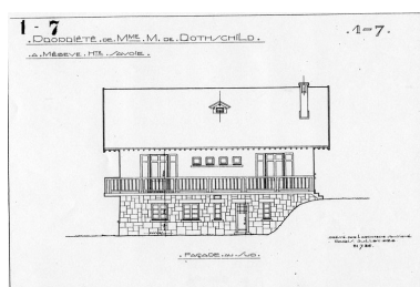
Elévation sud / Henri Jacques Le Même, 31 juillet 1926 Phot. F. Véry, Autr. Le Même Henry Jacques (architecte) IVR82_20127402167NUC
