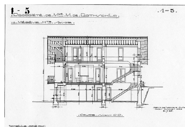
Coupe transversale / Henri Jacques Le Même, 31 juillet 1926 Phot. F. Véry, Autr. Le Même Henry Jacques (architecte) IVR82_20127402165NUC
