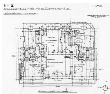
Plan du bel étage (rez-de- chaussée surélevé) / Henri Jacques Le Même, 31 juillet 1926 Phot. F. Véry, Autr. Le Même Henry Jacques (architecte) IVR82_20127402162NUC
