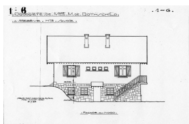
Elévation nord / Henri Jacques Le Même, 31 juillet 1926 Phot. F. Véry, Autr. Le Même Henry Jacques (architecte) IVR82_20127402166NUC
