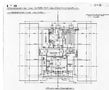
Plan des combles / Henri Jacques Le Même, 31 juillet 1926 Phot. F. Véry, Autr. Le Même Henry Jacques (architecte) IVR82_20127402163NUC
