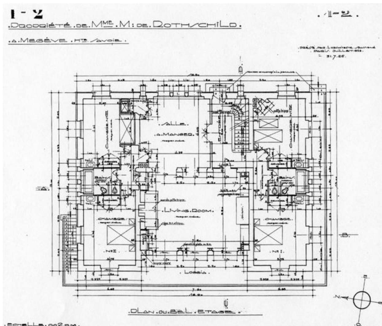
Plan du bel étage (rez-de-chaussée surélevé) / Henri Jacques Le Même, 31 juillet 1926
