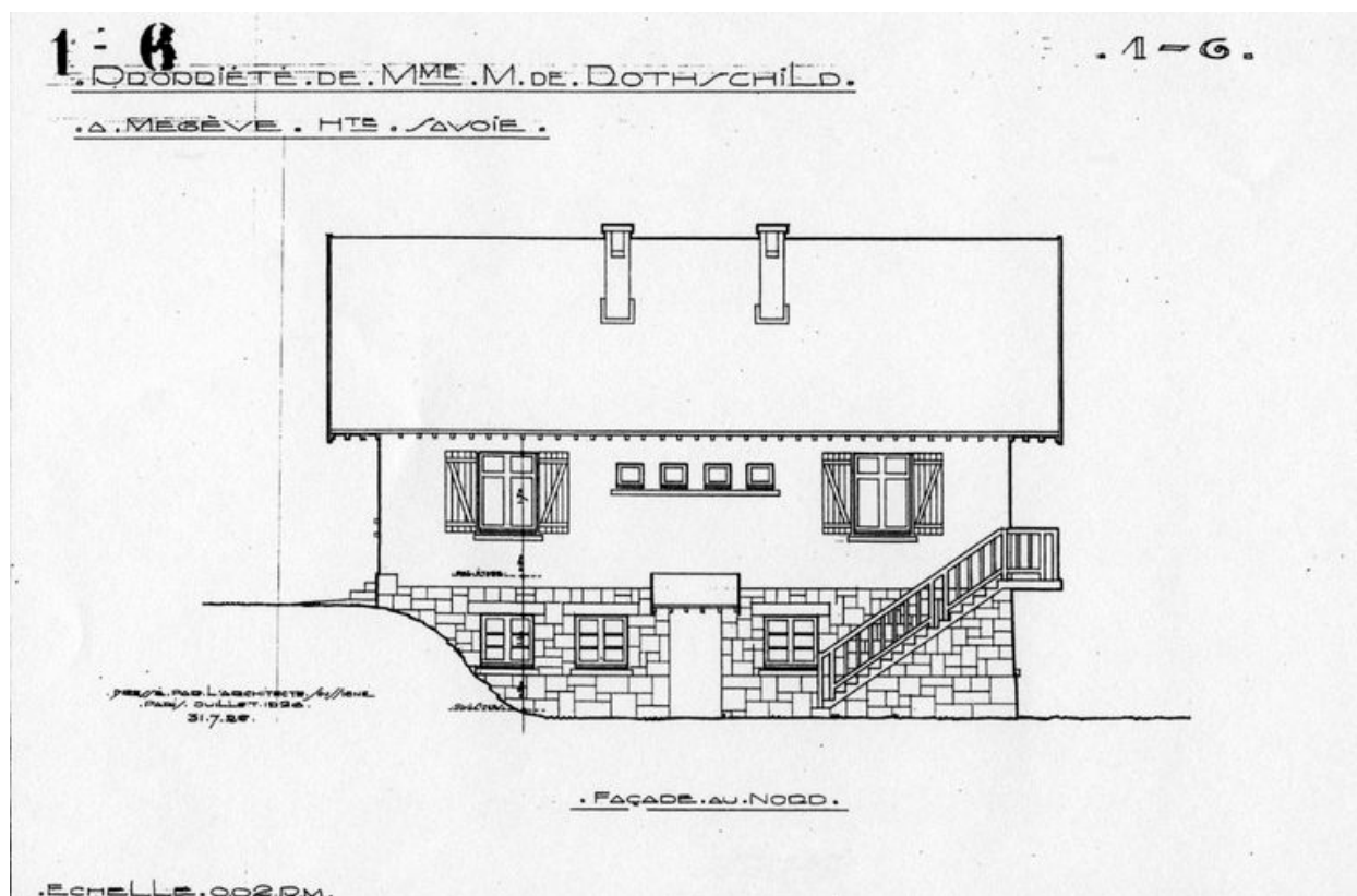
Elévation nord / Henri Jacques Le Même, 31 juillet 1926
