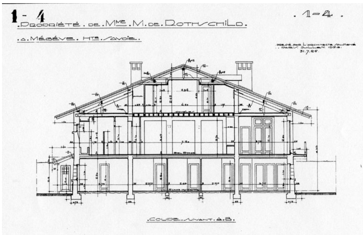
Coupe longitudinale / Henri Jacques Le Même, 31 juillet 1926
