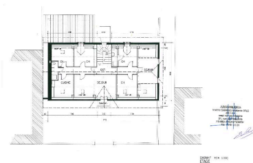
Plan, étage Repr. Denys Harreau IVR84_20167300061NUCB
