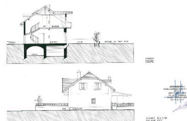
Coupe et élévation est Repr. Denys Harreau IVR84_20167300062NUCB
