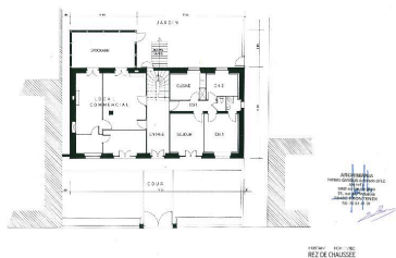
Plan, rez-de-chaussée Repr. Denys Harreau IVR84_20167300060NUCB
