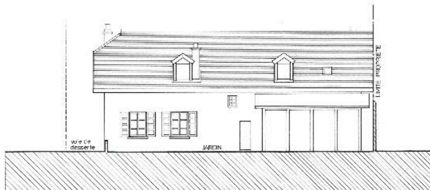
EXISTANT ECH. 1/100 FACADE NORD FACADE SUR JARDIN
