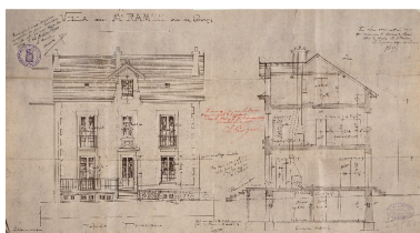
Coupe et élévation Repro. François Fouger IVR82_20097301241NUCB
