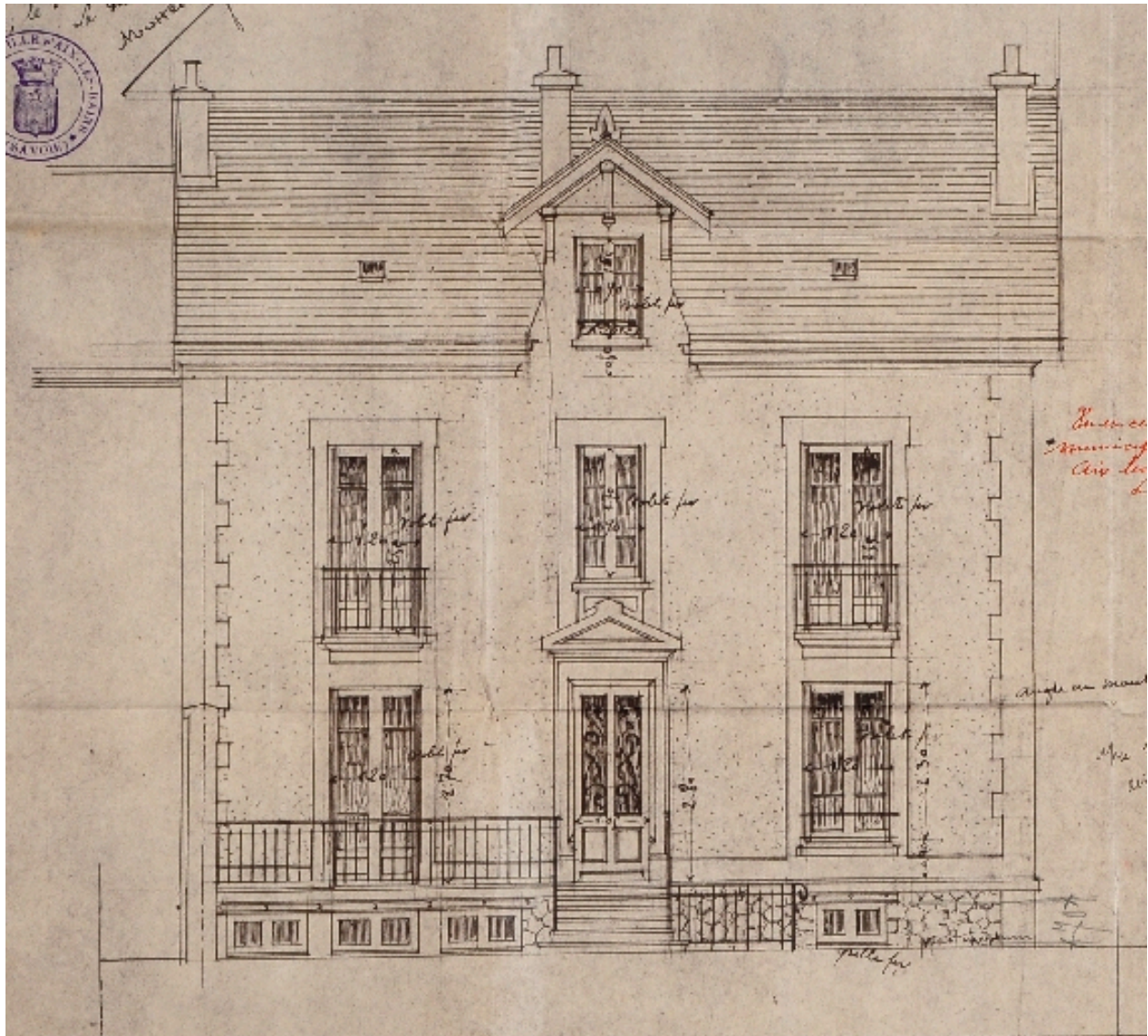
Elévation principale
