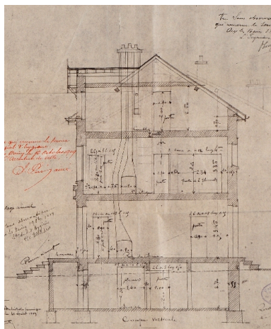
Coupe Repro. François Fouger IVR82_20097301242NUCB
