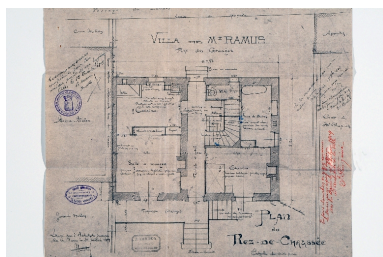
Plan du rez-de-chaussée Repro. François Fouger IVR82_20097301042NUCB
