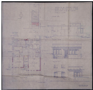
Plans, coupe et élévation, 1948 Repro. Denys Harreau IVR82_20137300505NUCB
