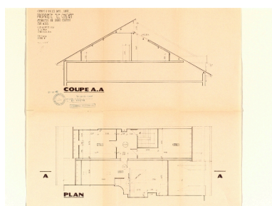
Plan et coupe des combles Repro. François Fouger IVR82_20057302014NUCB
