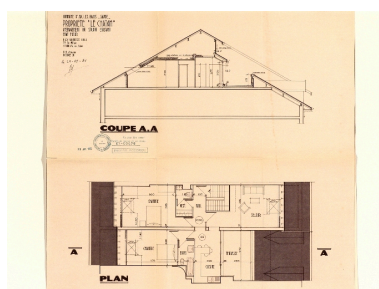
Projet d'aménagement des combles Repro. François Fouger IVR82_20057302015NUCB
