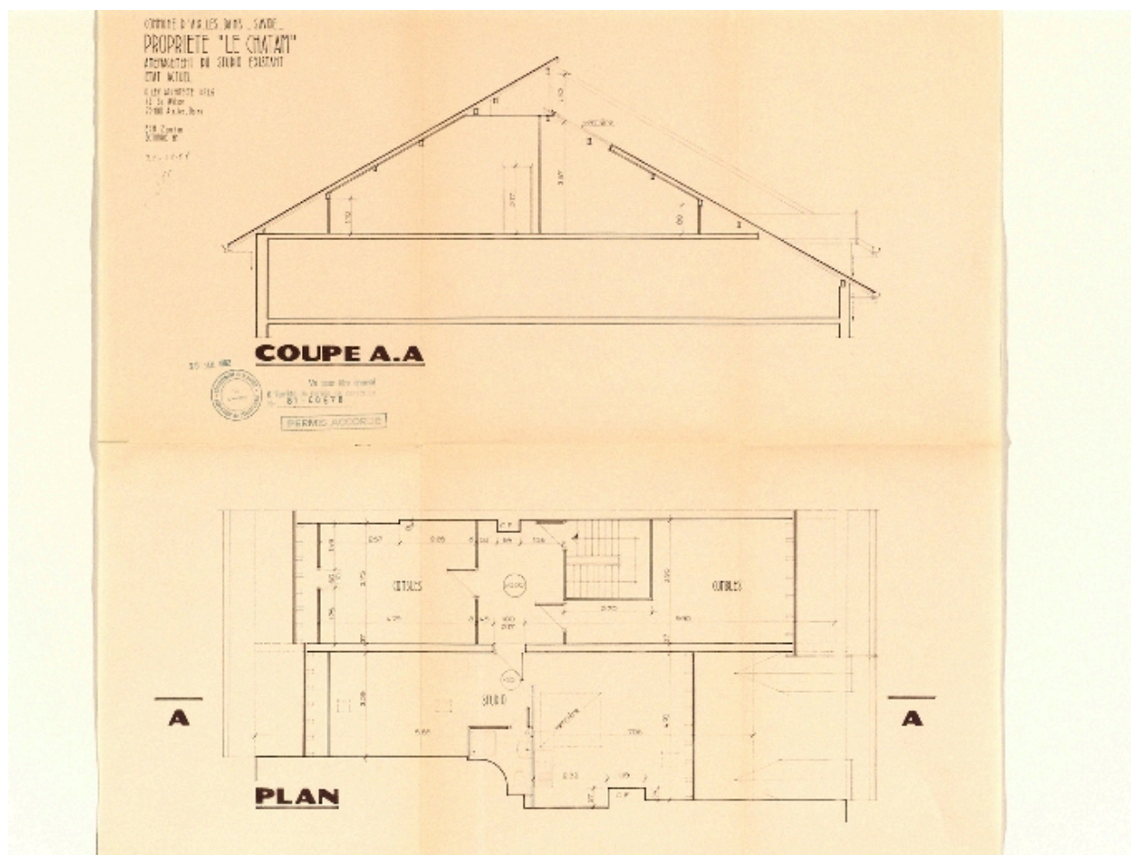
Plan et coupe des combles
