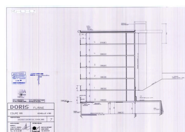
Coupe AA. M.B. A architectes, SCPA Jossa-Chiquet-Loehr-Michaelles-Vallejos, SOBATIM maître d'oeuvre, 3 avril 1989 (AC Arâches-la-Frasse)
