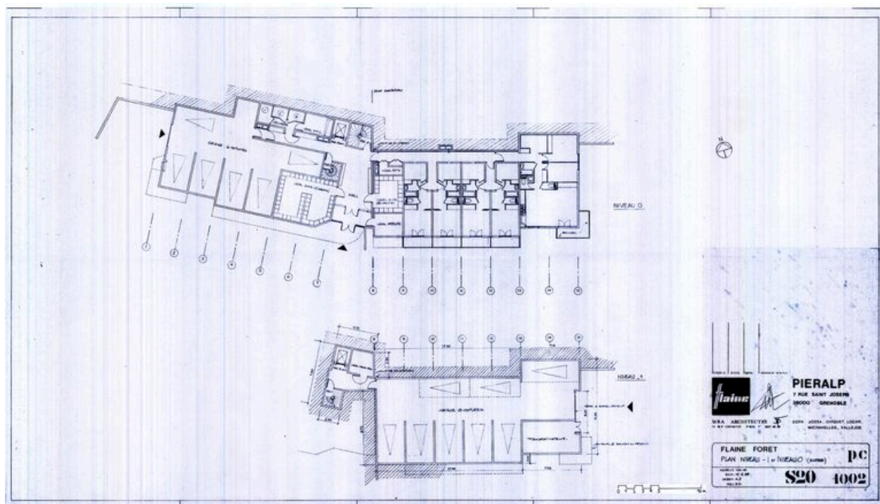
Plan des niveaux -1 et 0 (entrée). M.B. A architectes, SCPA Jossa-Chiquet-Loehr-Michaelles-Vallejos, 15 décembre 1988 (AC Arâches-la-Frasse)
