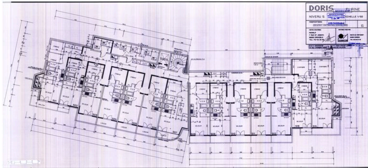
Plan niveau 5. M.B. A architectes, SCPA Jossa-Chiquet-Loehr-Michaelles-Vallejos, SOBATIM maître d'oeuvre, 3 avril 1989 (AC Arâches-la-Frasse)
