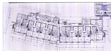
Plan niveau 3. M.B. A architectes, SCPA Jossa-Chiquet-Loehr-Michaelles-Vallejos, SOBATIM maître d'oeuvre, 3 avril 1989 (AC Arâches-la-Frasse)
