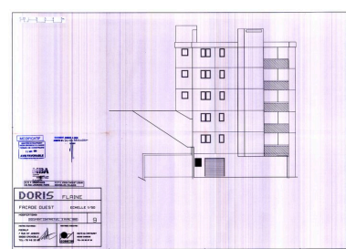
Elévation ouest. M.B. A architectes, SCPA Jossa-Chiquet-Loehr-Michaelles-Vallejos, SOBATIM maître d'oeuvre, 3 avril 1989 (AC Arâches-la-Frasse)
