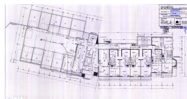
Plan niveau 0. M.B. A architectes, SCPA Jossa-Chiquet-Loehr-Michaelles-Vallejos, SOBATIM maître d'oeuvre, 3 avril 1989 (AC Arâches-la-Frasse) Phot. Jean-François Lyon-Caen, Phot. C. Salomon-Pelen, Autr. M.B.A. (agence d'architecture), Autr. SCPA Jossa-Chiquet-Loehr-Michaelles-Vallejos (agence d'architecture) IVR82_20117401963NUC
