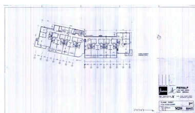
Plan des étages courants. M.B. A architectes, SCPA Jossa-Chiquet-Loehr-Michaelles-Vallejos, 15 décembre 1988 (AC Arâches-la-Frasse) Phot. Jean-François Lyon-Caen, Phot. C. Salomon-Pelen, Autr. M.B.A. (agence d'architecture), Autr. SCPA Jossa-Chiquet-Loehr-Michaelles-Vallejos (agence d'architecture) IVR82_20117401960NUC
