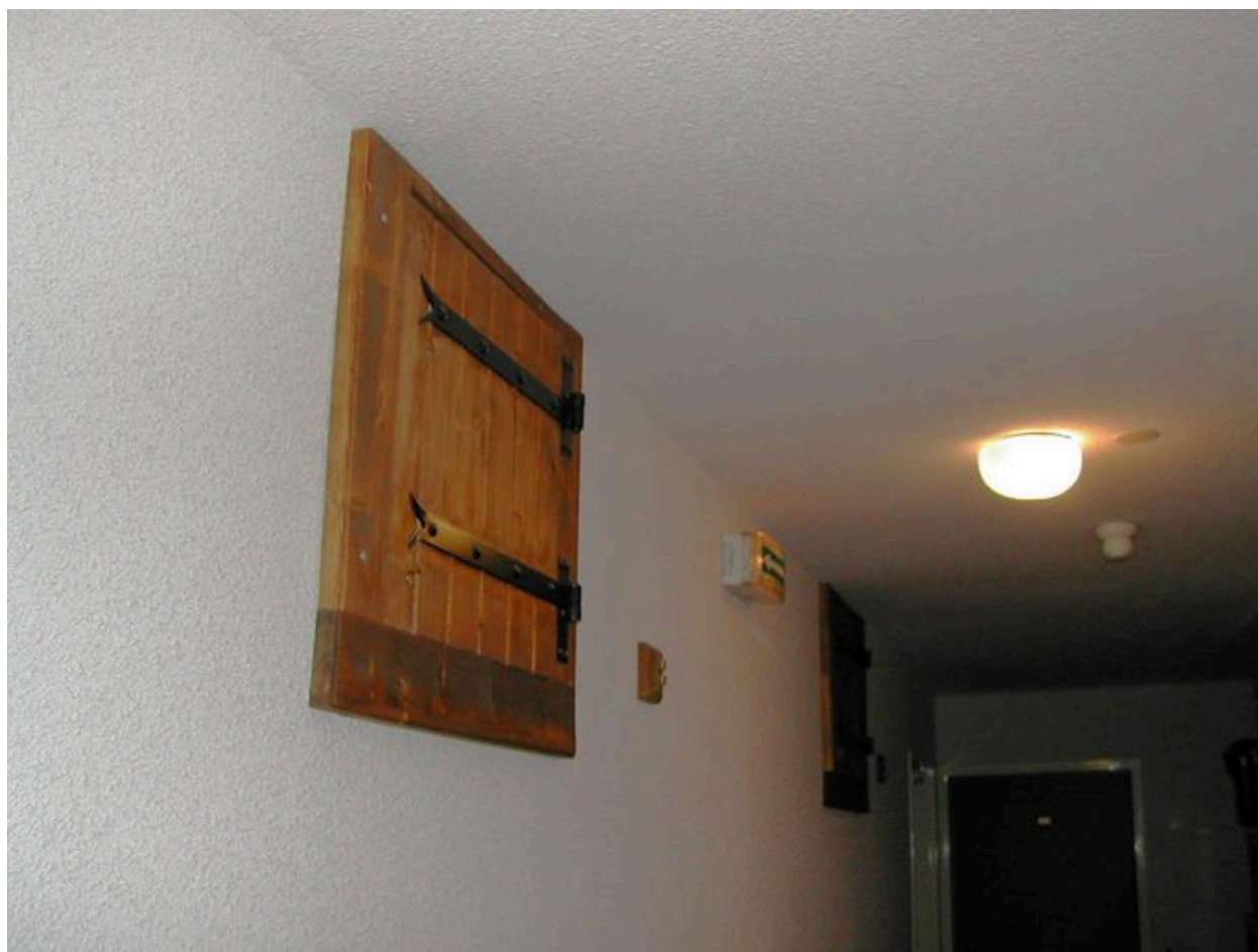
Fenêtre de second jour ouvrant sur le couloir de distribution des appartements
