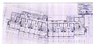
Plan niveau 4. M.B. A architectes, SCPA Jossa-Chiquet-Loehr-Michaelles-Vallejos, SOBATIM maître d'oeuvre, 3 avril 1989 (AC Arâches-la-Frasse)
