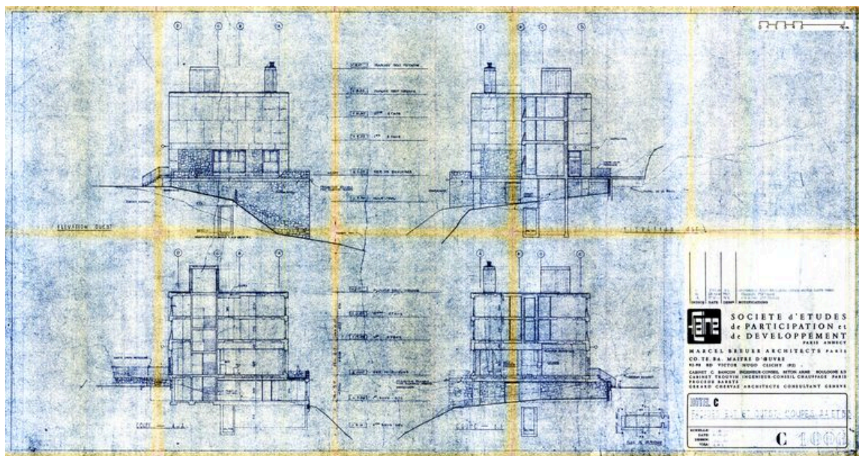
Hôtel C. Elévations est et ouest. Coupes transversales. Marcel Breuer architecte, 30 octobre 1967. Modification 7 février 1968 (AC Arâches-la-Frasse)
