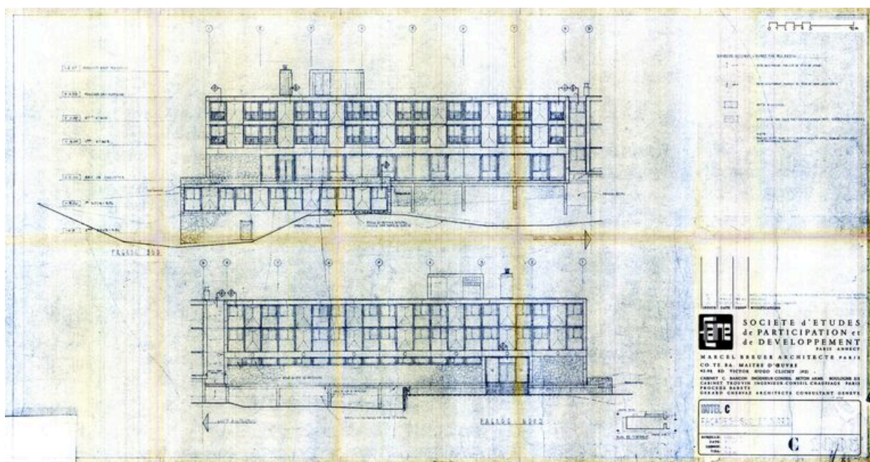
Hôtel C. Elévations sud et nord. Marcel Breuer architecte, 30 octobre 1967. Modification 7 février 1968 (AC Arâches-la-Frasse)
