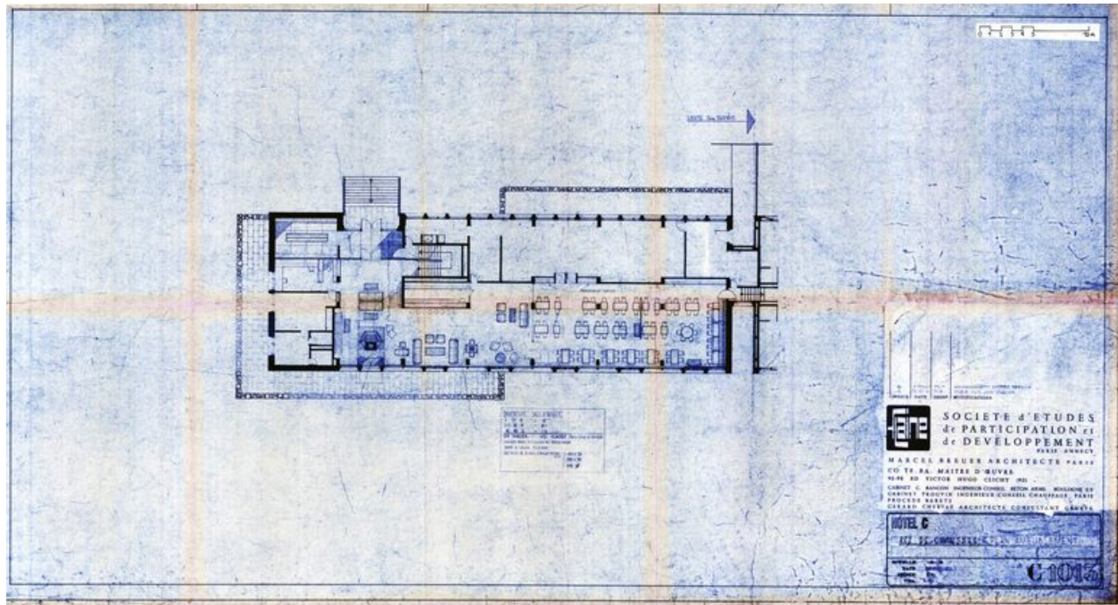
Hôtel C. Plan de l'ameublement du rez-de-chaussée. Marcel Breuer architecte, 30 octobre 1967 (AC Arâches-la-Frasse)
