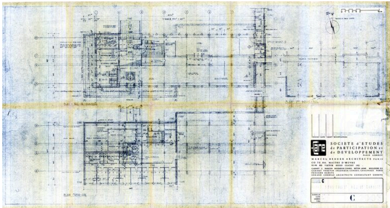
Hôtel C. Plans du sous-sol et du rez-de-chaussée. Marcel Breuer architecte, 30 octobre 1967. Modification 7 février 1968 (AC Arâches-la-Frasse)
