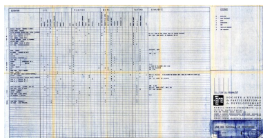
Hôtel C. Liste des matériaux de revêtement. Marcel Breuer architecte, 30 octobre 1967. Modification 7 février 1968 (AC Arâches-la-Frasse)
