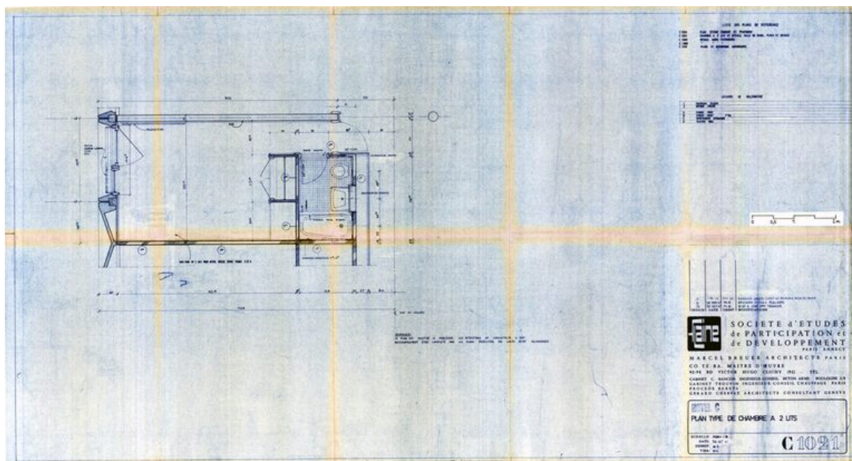
Hôtel C. Plan type d'une chambre à 2 lits. Marcel Breuer architecte, 30 octobre 1967. Modification 7 février 1968 (AC Arâches-la-Frasse)
