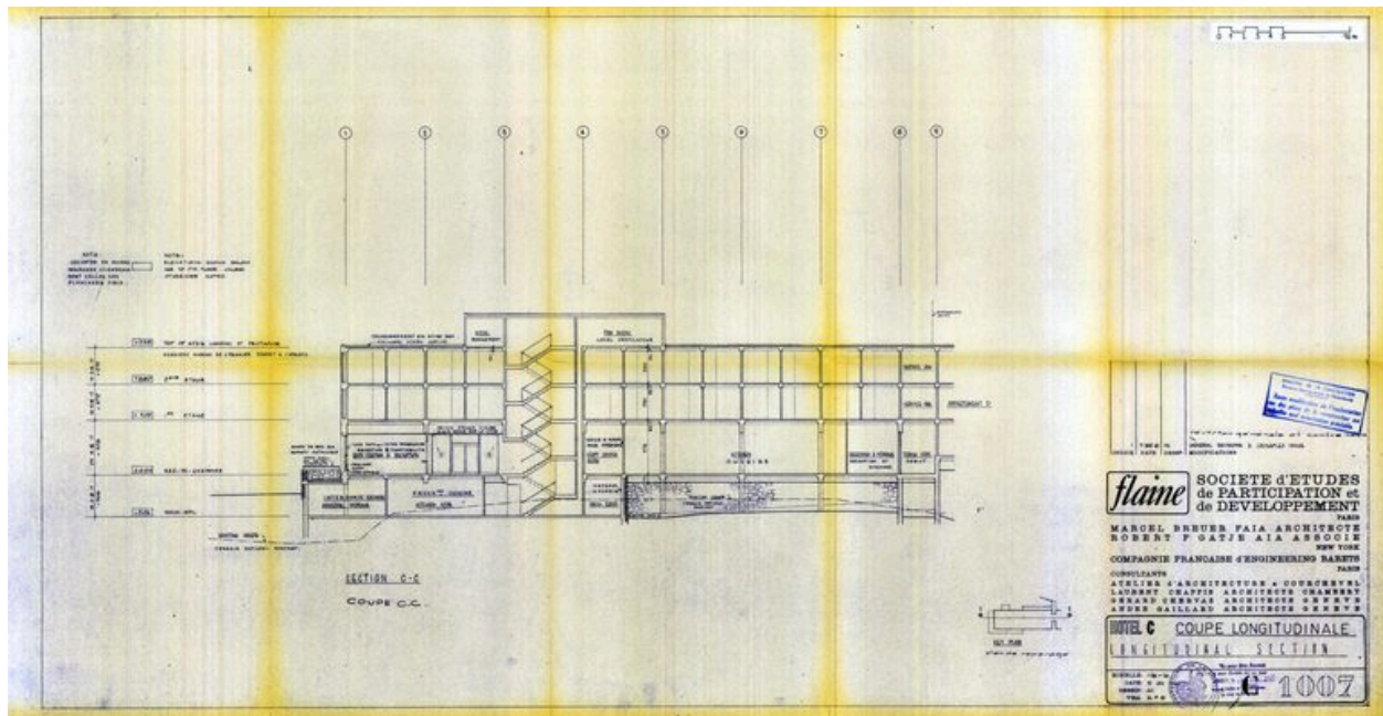
Hôtel C. Coupe longitudinale. Marcel Breuer architecte, Robert F. Gatje associé, 31 janvier 1962 (AC Arâches-la-Frasse)
