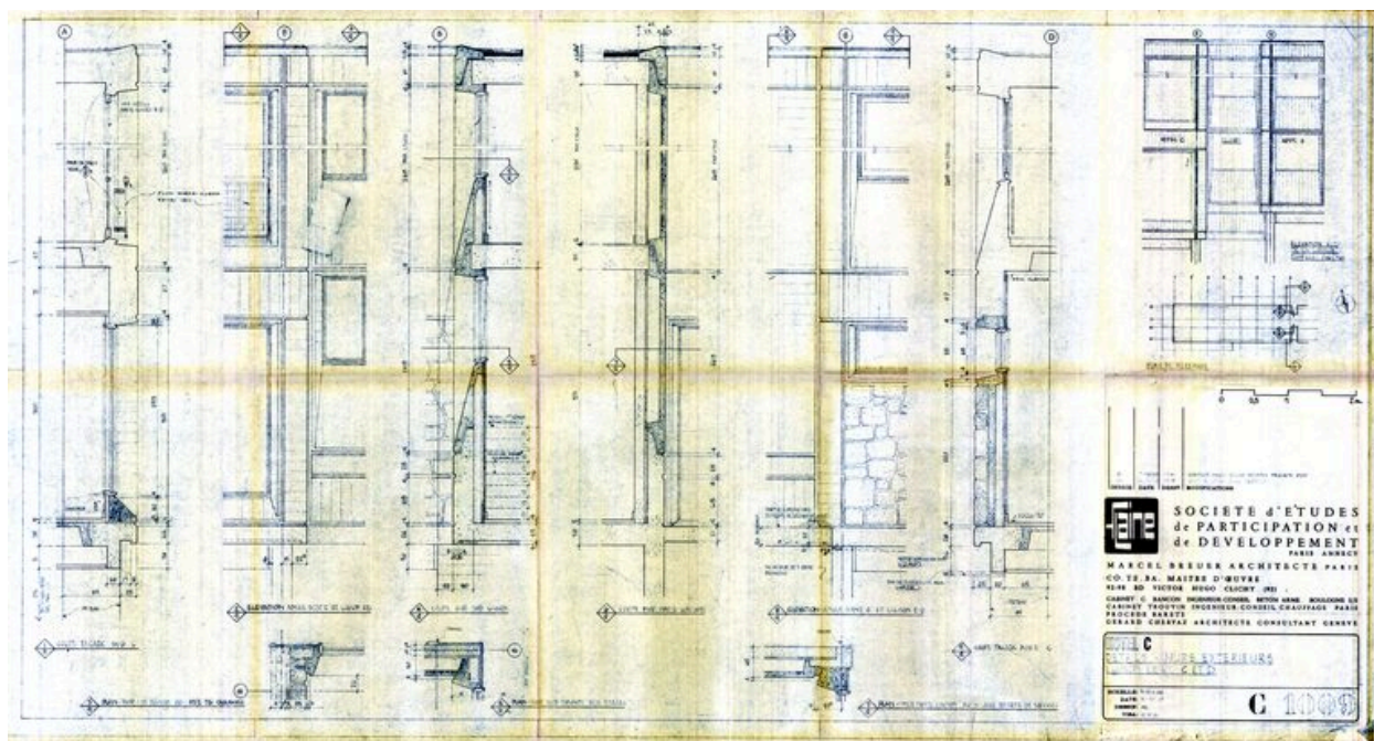
Hôtel C. Détails des murs extérieurs. Liaison entre C et D. Marcel Breuer architecte, 30 octobre 1967. Modification 7 février 1968 (AC Arâches-la-Frasse)
