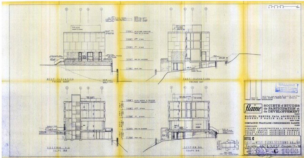
Hôtel C. Elévations est et ouest. Coupes transversales. Marcel Breuer architecte, Robert F. Gatje associé, 31 janvier 1962 (AC Arâches-la-Frasse)
