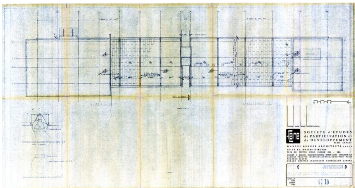
Hôtel C. Appartement D. Projection du plafond des étages. Plans et détails. Marcel Breuer architecte, 30 octobre 1967 (AC Arâches-la-Frasse)
