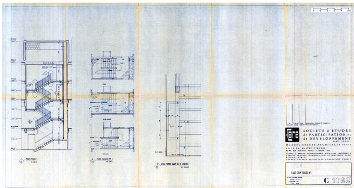
Hôtel C. Plans et coupe de l'escalier n° 1. Marcel Breuer architecte, 5 décembre 1967 (AC Arâches-la-Frasse)
