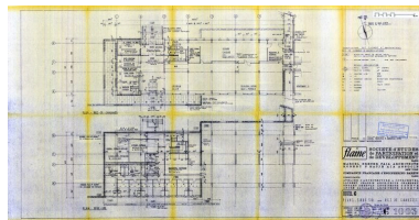
Hôtel C. Plans des sous-sol et rez-de-chaussée. Marcel Breuer architecte, Robert F. Gatje associé, 31 janvier 1962 (AC Arâches-la-Frasse) Phot. Jean-François Lyon-Caen, Phot. C. Salomon-Pelen, Autr. Breuer Marcel (architecte), Autr. Gatje Robert F. (architecte) IVR82_20117402318NUC
