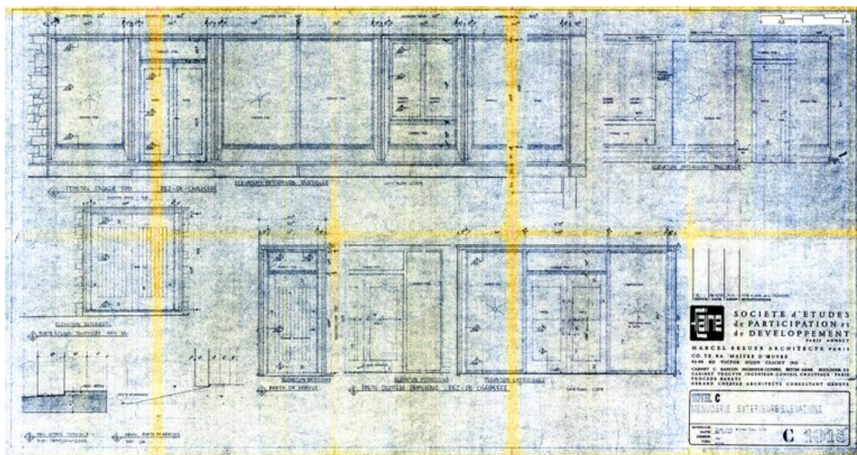
Hôtel C. Détails des menuiseries extérieures. Marcel Breuer architecte, 30 octobre 1967 (AC Arâches-la-Frasse)
