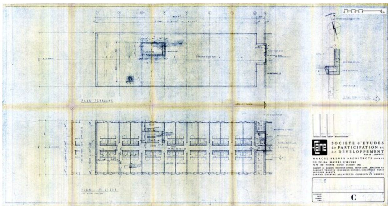
Hôtel C. Plans d'un étage courant et du toit-terrasse. Marcel Breuer architecte, 30 octobre 1967 (AC Arâches-la-Frasse)
