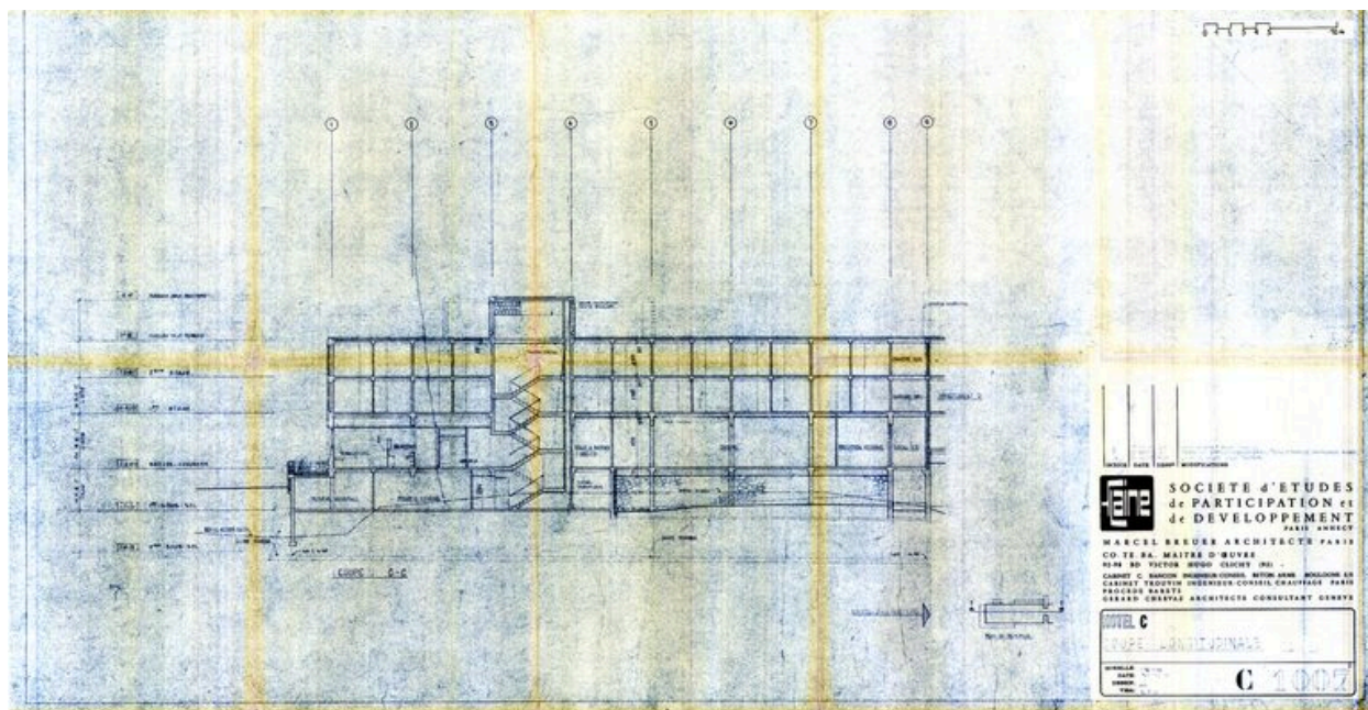
Hôtel C. Coupe longitudinale. Marcel Breuer architecte, 30 octobre 1967. Modification 7 février 1968 (AC Arâches-la-Frasse)
