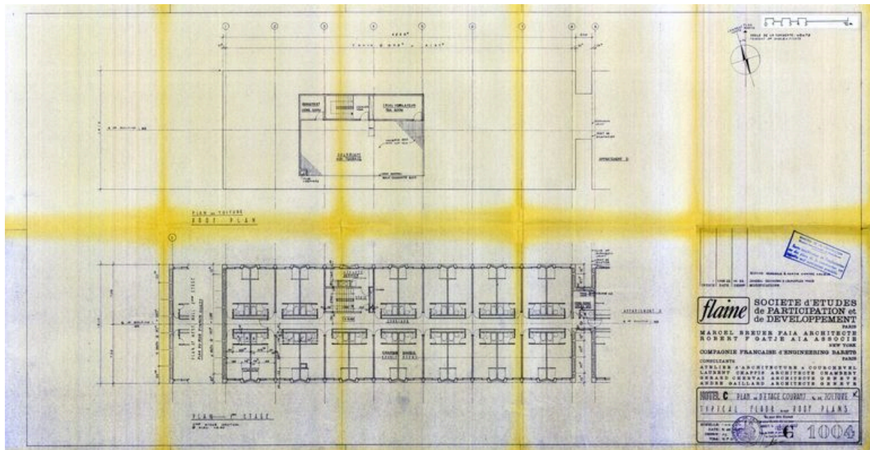
Hôtel C. Plans de l'étage courant et de toiture. Marcel Breuer architecte, Robert F. Gatje associé, 31 janvier 1962 (AC Arâches-la-Frasse)
