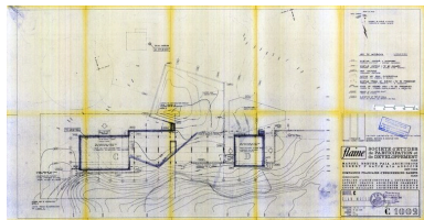
Hôtel C. Plan masse. Marcel Breuer architecte, Robert F. Gatje associé, 31 janvier 1962 (AC Arâches-la-Frasse) Phot. Jean-François Lyon-Caen, Phot. C. Salomon-Pelen, Autr. Breuer Marcel (architecte), Autr. Gatje Robert F. (architecte) IVR82_20117402317NUC
