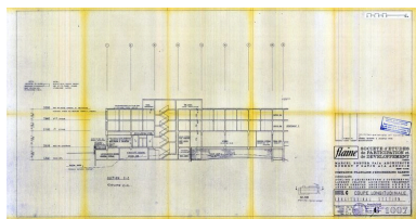
Hôtel C. Coupe longitudinale. Marcel Breuer architecte, Robert F. Gatje associé, 31 janvier 1962 (AC Arâches-la-Frasse) Phot. Jean-François Lyon-Caen, Phot. C. Salomon-Pelen, Autr. Breuer Marcel (architecte), Autr. Gatje Robert F. (architecte) IVR82_20117402320NUC
