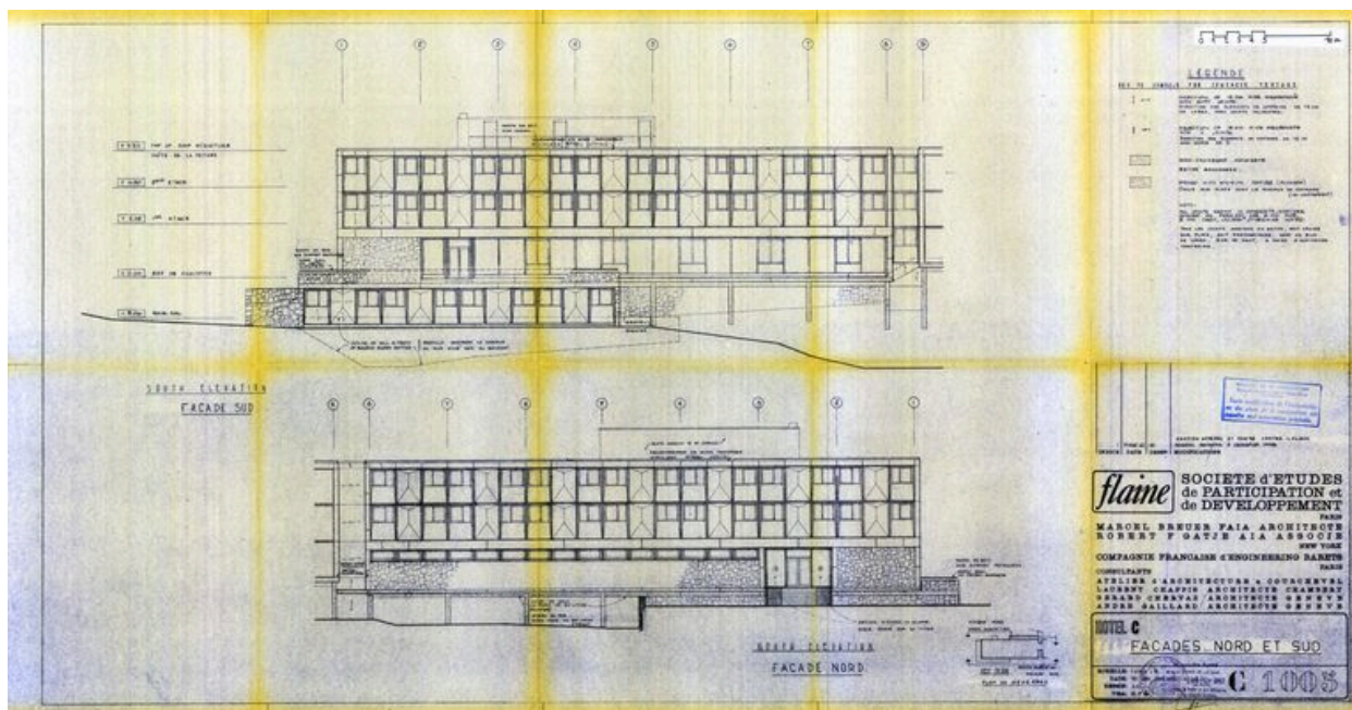
Hôtel C. Elévations nord et sud. Marcel Breuer architecte, Robert F. Gatje associé, 31 janvier 1962 (AC Arâches-la-Frasse)
