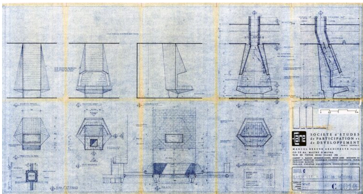
Hôtel C. Plans, coupes et élévations de la cheminée du rez-de-chaussée. Marcel Breuer architecte, 30 octobre 1967 (AC Arâches-la-Frasse)
