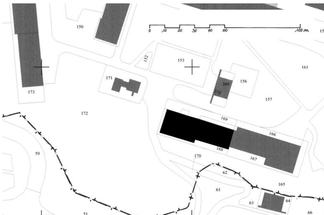
Plan masse, d'après le plan cadastral d'Arâches-la-Frasse, section CO1, 2006
