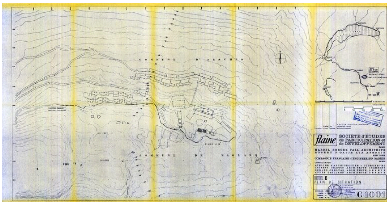
Hôtel C. Plan de situation. Marcel Breuer architecte, Robert F. Gatje associé, 31 janvier 1962 (AC Arâches-la-Frasse)
