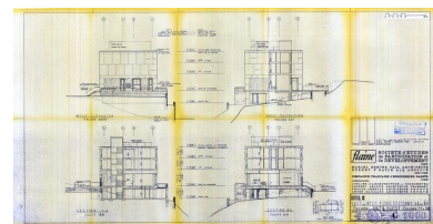
Hôtel C. Elévations est et ouest. Coupes transversales. Marcel Breuer architecte, Robert F. Gatje associé, 31 janvier 1962 (AC Arâches-la-Frasse) Phot. Jean-François Lyon-Caen, Phot. C. Salomon-Pelen, Autr. Breuer Marcel (architecte), Autr. Gatje Robert F. (architecte) IVR82_20117402322NUC
