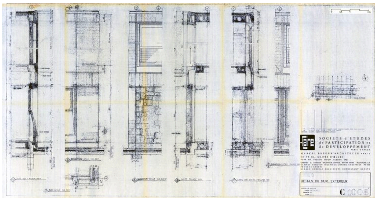
Hôtel C. Détails du mur extérieur. Façade sud. Marcel Breuer architecte, 30 octobre 1967. Modification 7 février 1968 (AC Arâches-la-Frasse)
