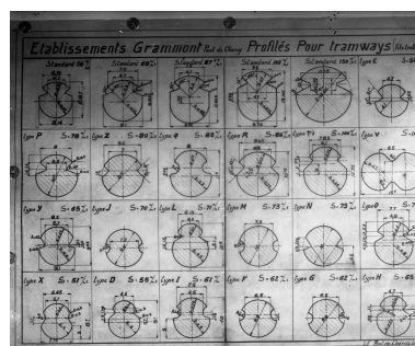
Planche de dessins techniques de profilés pour tramways, AD 69 : série 158 J. usine Tréfinétaux AD Rhône. 158 J Repro. Nadine Halitim-Dubois IVR82_20093800775NUCB
