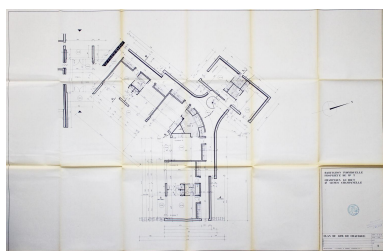
Saint-Genès-Champanelle, la Maison T., plan du rez-de-chaussée, partie "enfants" (version du permis de construire), 1970, Jean-François Cousin et Aimé Vernay architectes (Archives municipales de Saint-Genès-Champanelle). Repro. Christophe Laurent, Autr. Jean-François COUSIN, Autr. Aimé Vernay IVR84_20216302485NUCA
