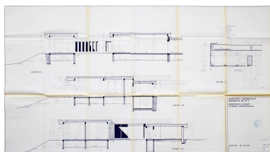
Saint-Genès-Champanelle, la Maison T., coupes AB, CD, EF (version du permis de construire), 1970, Jean-François Cousin et Aimé Vernay architectes (Archives municipales de Saint-Genès-Champanelle). Repro. Christophe Laurent, Autr. Jean-François COUSIN, Autr. Aimé Vernay IVR84_20216302488NUCA
