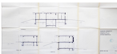
Saint-Genès-Champanelle, la Maison T., coupes GH, IJ, KF (version du permis de construire), 1970, Jean-François Cousin et Aimé Vernay architectes (Archives municipales de Saint-Genès-Champanelle). Repro. Christophe Laurent, Autr. Jean-François COUSIN, Autr. Aimé Vernay IVR84_20216302489NUCA
