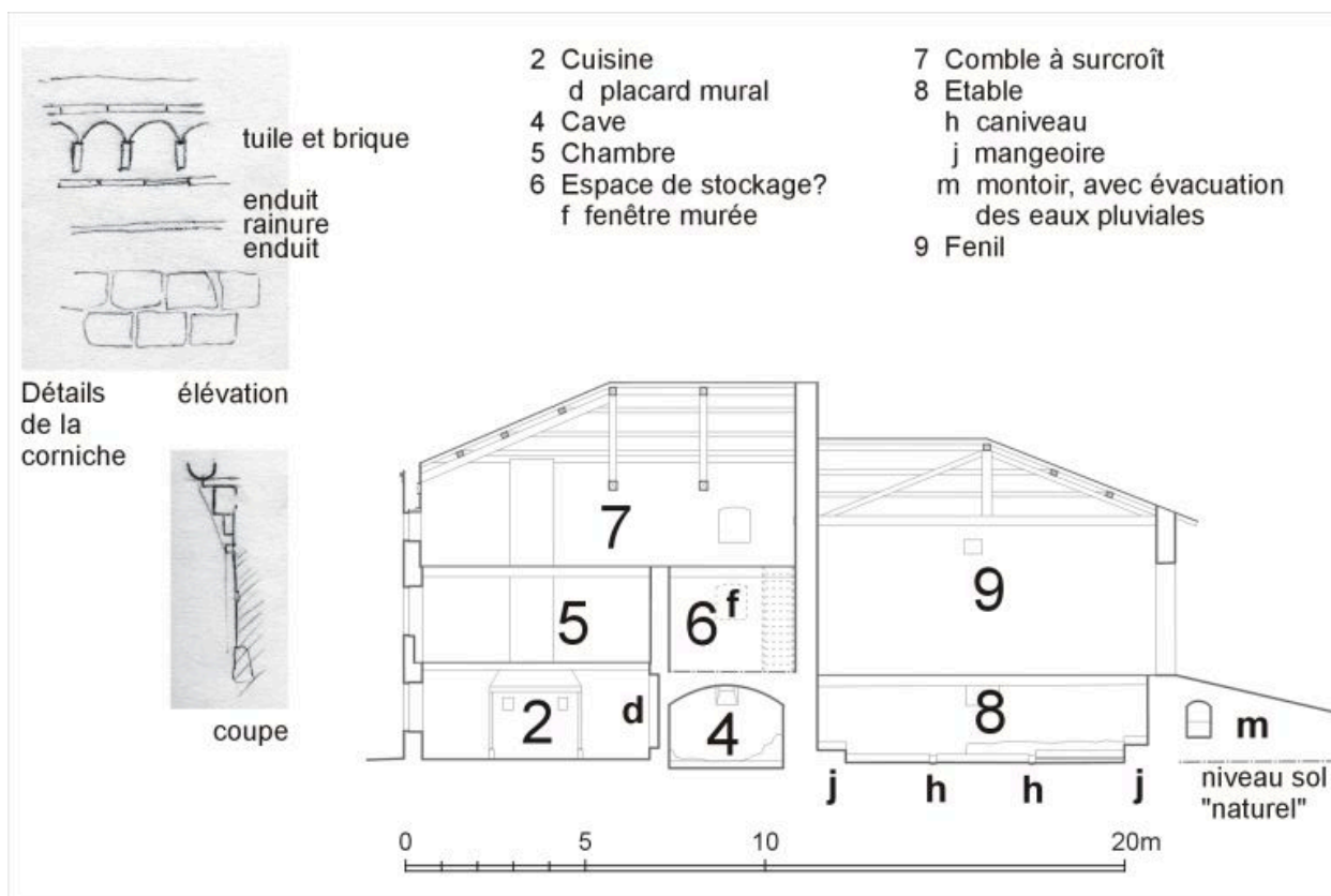
Coupe XX'. Relevé manuel expédié. Détails de la corniche. Croquis.
