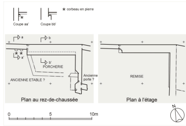
Vestige d'un bâtiment primitif. Plan au rez-de-chaussée. Plan à l'étage. Relevés manuels expédiés et schématiques. Dess. Paul Cherblanc, Dess. S. Bassieux IVR82_20114201720NUD
