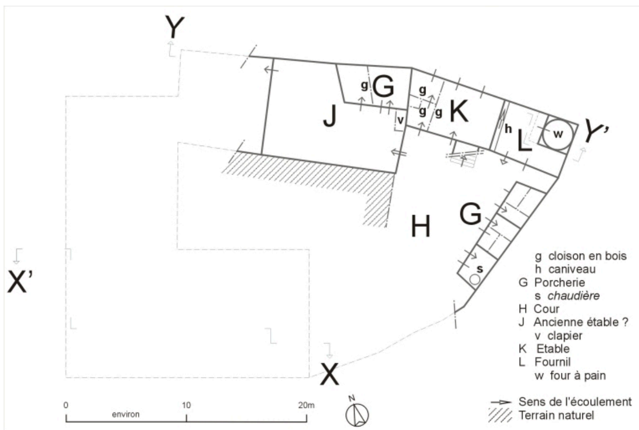
Plan de l'étage de soubassement. Schéma.
