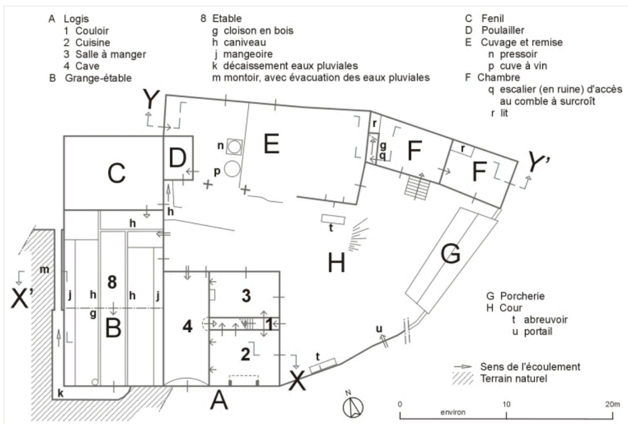
Plan du rez-de-chaussée surélevé. Schéma.
