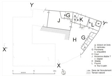
Plan de l'étage de soubassement. Schéma. Dess. Paul Cherblanc, Dess. S. Bassieux IVR82_20114201717NUD
