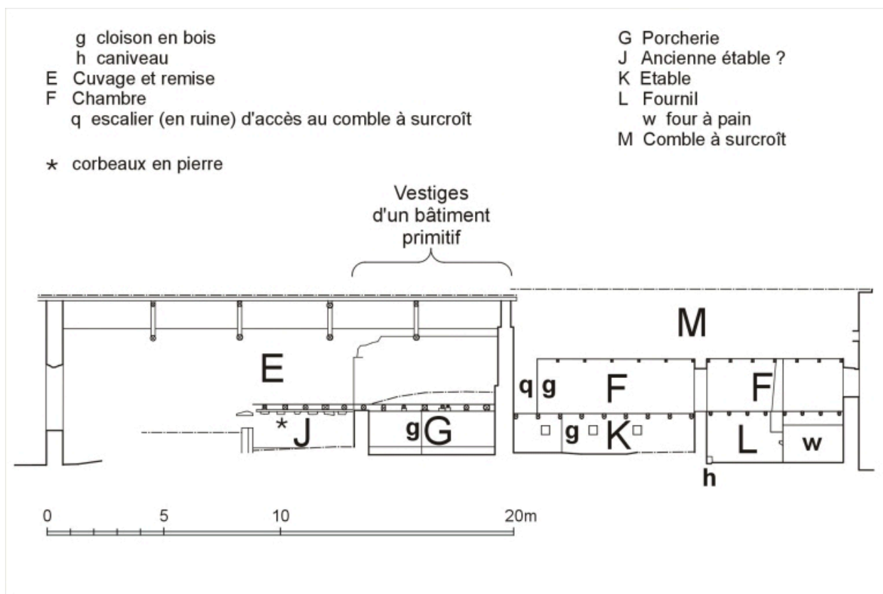
Coupe YY'. Relevé manuel expédié et schématique.
