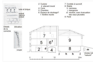
Coupe XX'. Relevé manuel expédié. Détails de la corniche. Croquis. Dess. Paul Cherblanc, Dess. S. Bassieux IVR82_20114201721NUD
