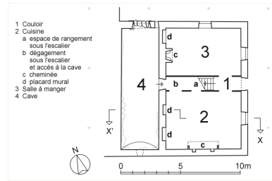
Logis. Plan du rez-de-chaussée. Relevé manuel expédié. Dess. Paul Cherblanc, Dess. S. Bassieux IVR82_20114201718NUD
