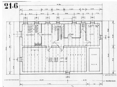
Plan de l'étage de soubassement. Henry Jacques Le Même [1928] Phot. F. Véry, Autr. Le Même Henry Jacques (architecte) IVR82_20127402115NUC
