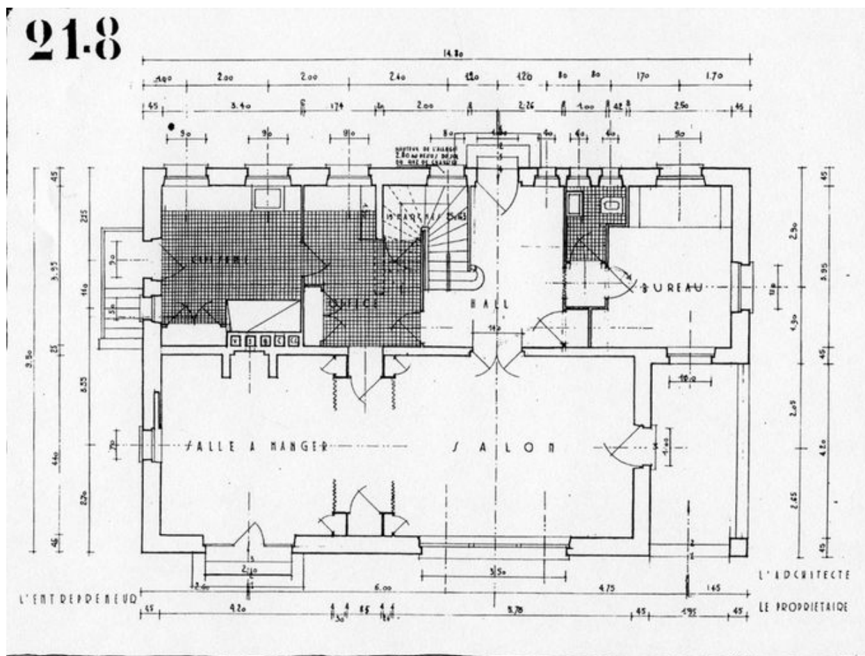
Plan du rez-de-chaussée surélevé. Henry Jacques Le Même [1928]
