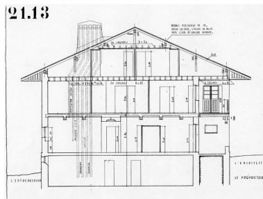
Coupe longitudinale. Henry Jacques Le Même [1928] Phot. F. Véry, Autr. Le Même Henry Jacques (architecte) IVR82_20127402120NUC
