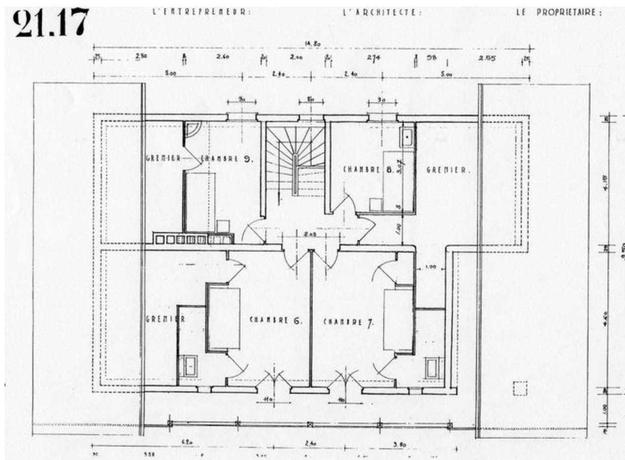
Plan de l'étage de comble. Henry Jacques Le Même [1928]
