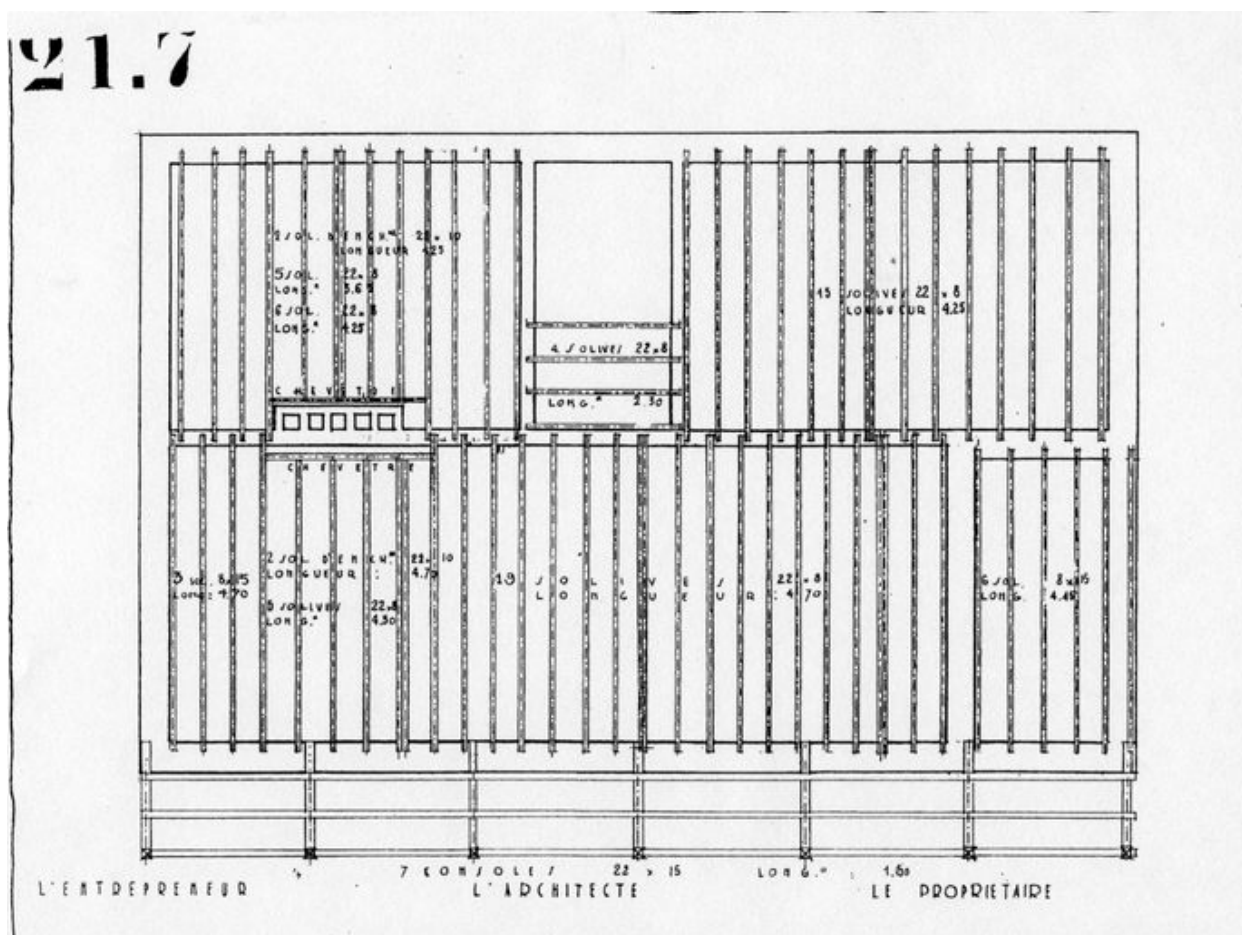
Plan de charpente. Henry Jacques Le Même [1928]
