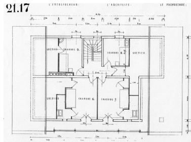
Plan de l'étage de comble. Henry Jacques Le Même [1928] Phot. F. Véry, Autr. Le Même Henry Jacques (architecte) IVR82_20127402123NUC
