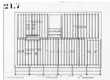
Plan de charpente. Henry Jacques Le Même [1928] Phot. F. Véry, Autr. Le Même Henry Jacques (architecte) IVR82_20127402116NUC
