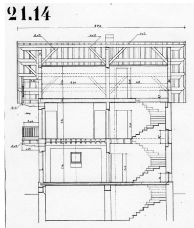
Coupe transversale. Henry Jacques Le Même [1928] Phot. F. Véry, Autr. Le Même Henry Jacques (architecte) IVR82_20127402121NUC
