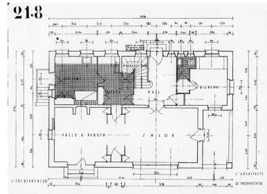
Plan du rez-de-chaussée surélevé. Henry Jacques Le Même [1928] Phot. F. Véry, Autr. Le Même Henry Jacques (architecte) IVR82_20127402117NUC
