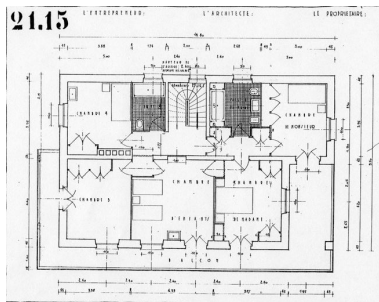
Plan de l'étage. Henry Jacques Le Même [1928] Phot. F. Véry, Autr. Le Même Henry Jacques (architecte) IVR82_20127402122NUC
