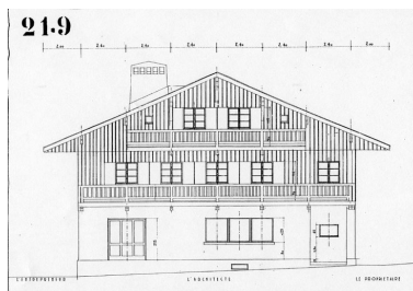
Elévation postérieure. Henry Jacques Le Même [1928] Phot. F. Véry, Autr. Le Même Henry Jacques (architecte) IVR82_20127402118NUC
