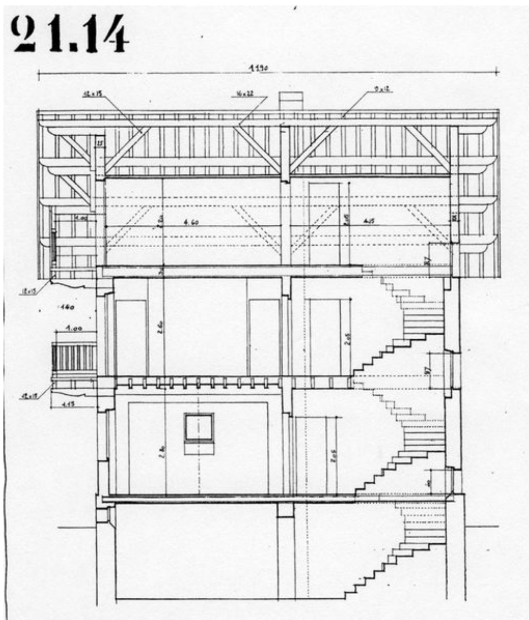
Coupe transversale. Henry Jacques Le Même [1928]
