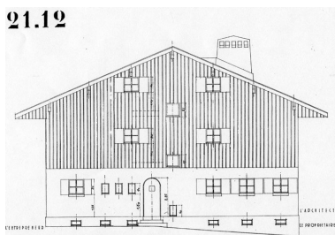
Elévation antérieure. Henry Jacques Le Même [1928] Phot. F. Véry, Autr. Le Même Henry Jacques (architecte) IVR82_20127402119NUC
