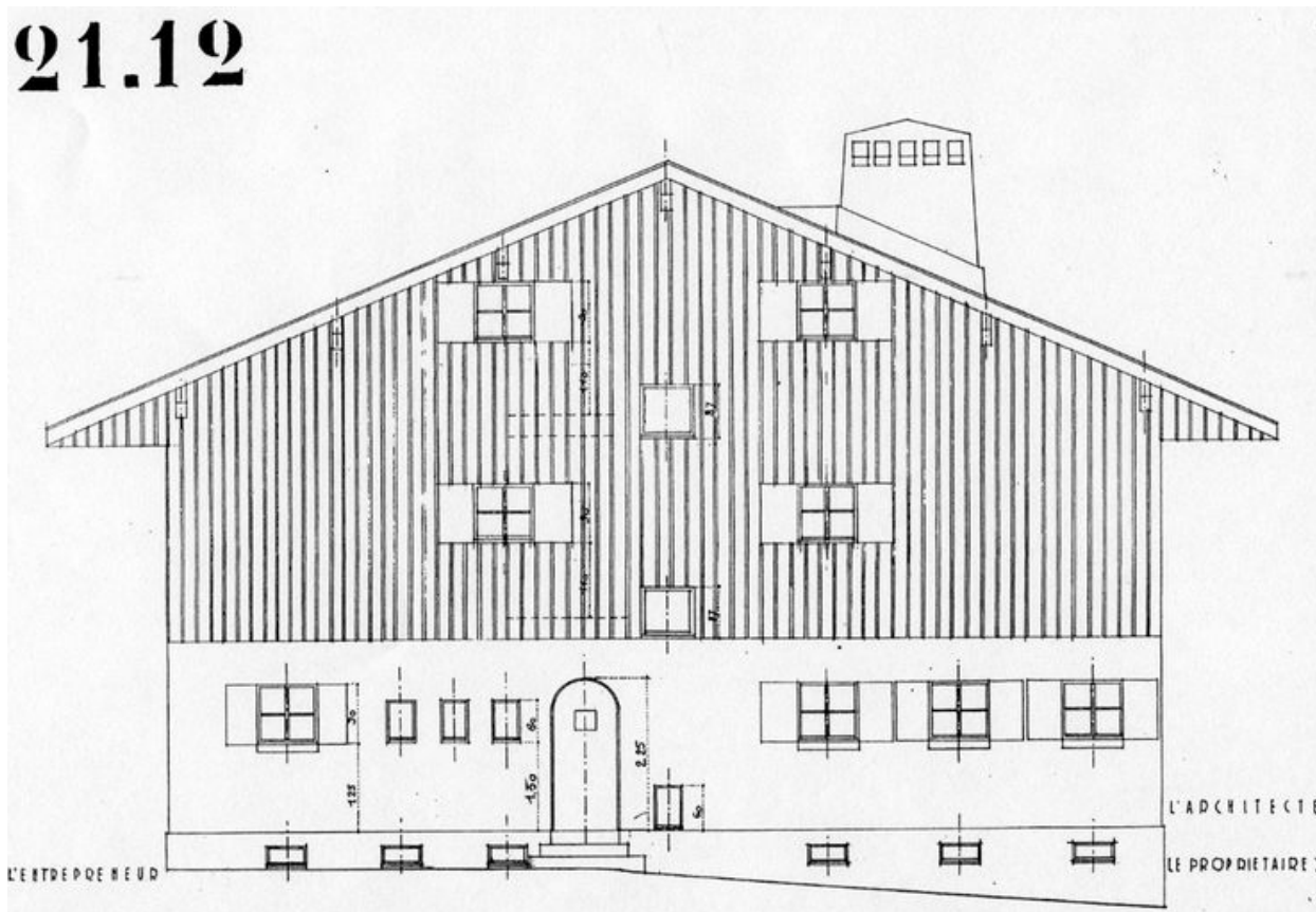
Elévation antérieure. Henry Jacques Le Même [1928]
