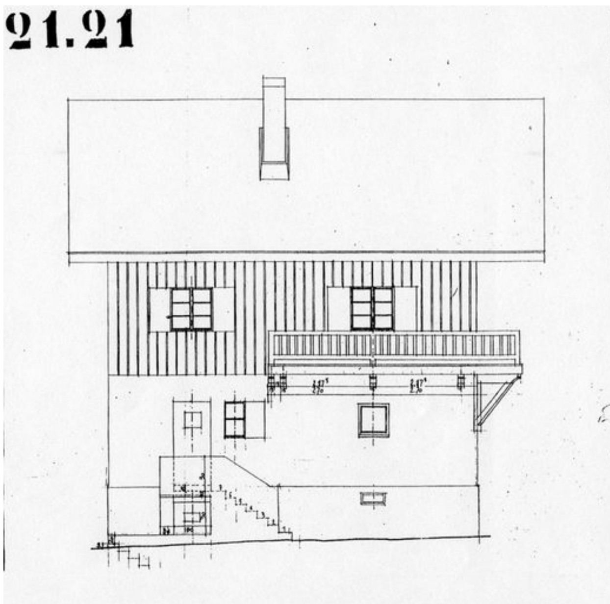
Elévation latérale. Henry Jacques Le Même [1928]
