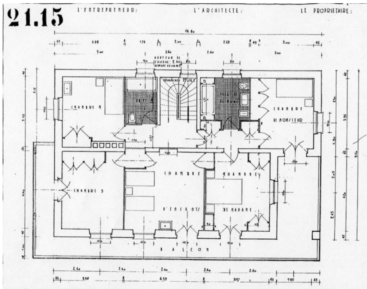
Plan de l'étage. Henry Jacques Le Même [1928]
