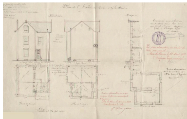
Plans, coupe et élévations, 1911 Repro. Denys Harreau IVR82_20137301017NUCB
