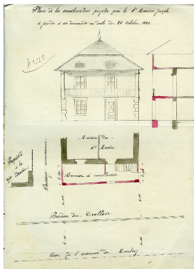
Agrandissement : plan, coupe et élévation Repro. François Fouger IVR82_20087300280NUCB
