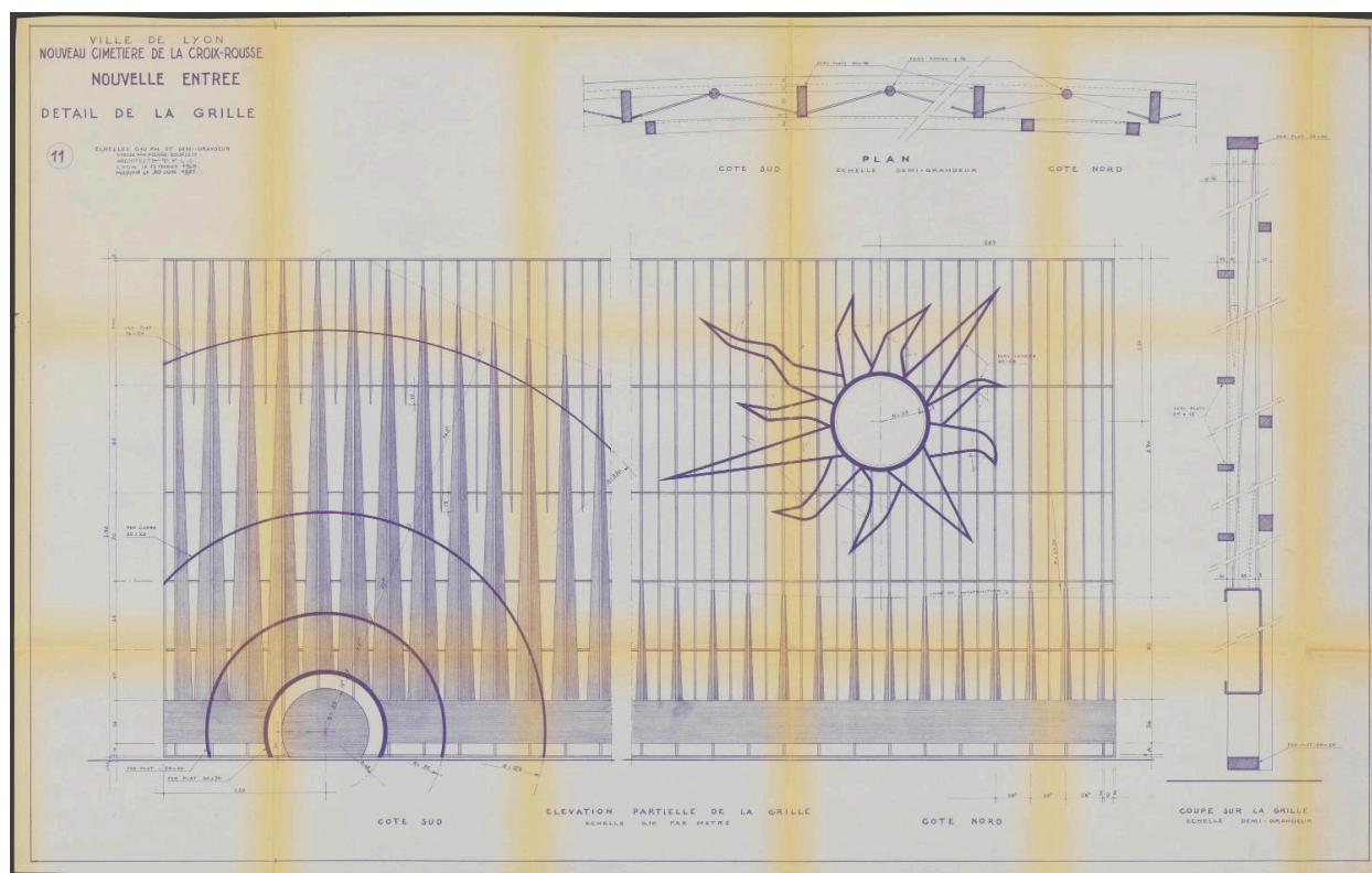
Détail de la grille : plan, coupe, élévations partielles, février 1968, modifié en juin 1971
