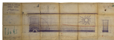
Grille et portillon, coupe, élévations : plan d'exécution, 1968-1971, annoté en 1972 Phot. Franck Trabouillet IVR84_20206901242NUCA
