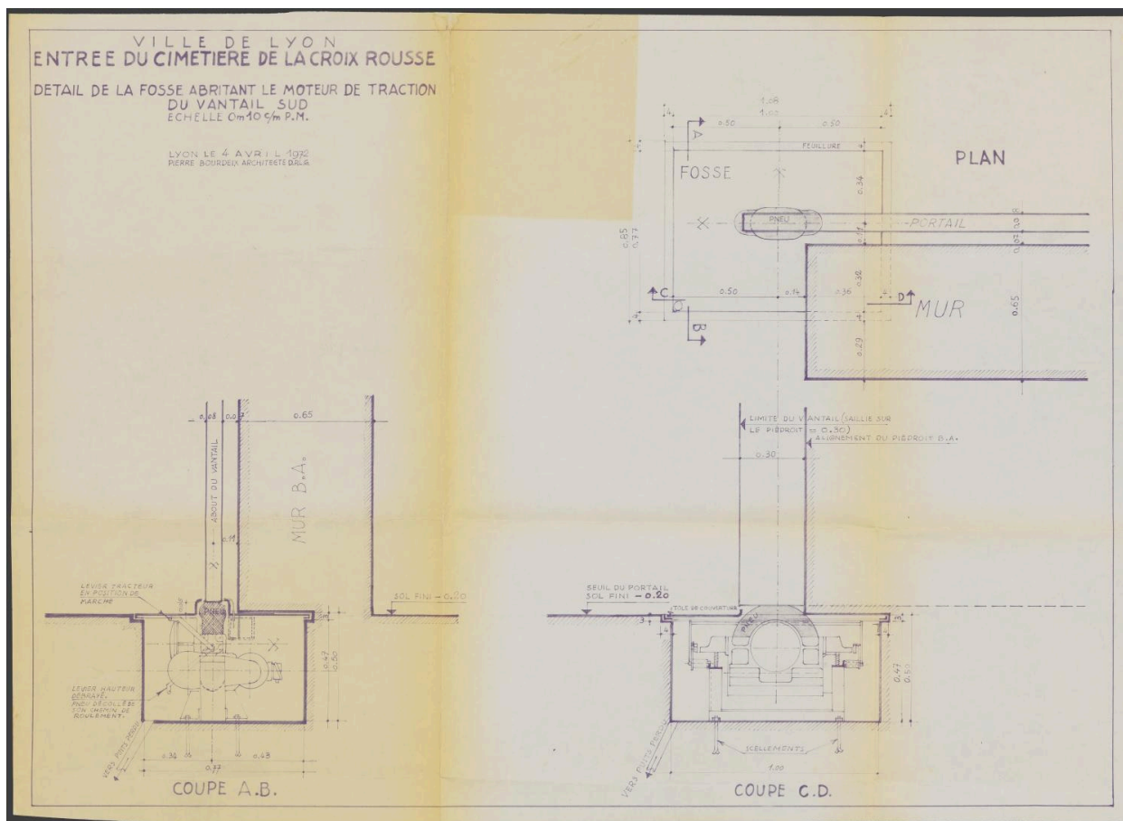
Détail de la fosse abritant le moteur de traction du vantail sud, plan, coupes, 1972
