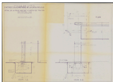
Détail de la fosse abritant le moteur de traction du vantail sud, plan, coupes, 1972 Repro. Gilles Bernasconi IVR84_20256901608NUCA
