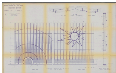
Détail de la grille : plan, coupe, élévations partielles, février 1968, modifié en juin 1971 Repro. Gilles Bernasconi IVR84_20256901637NUCA
