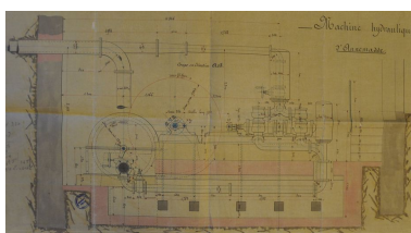
Coupe transversale de la machine hydraulique. Plan. Archives municipales d'Annemasse © Archives municipales d'Annemasse. 36/36 Phot. Samir Mahfoudi
