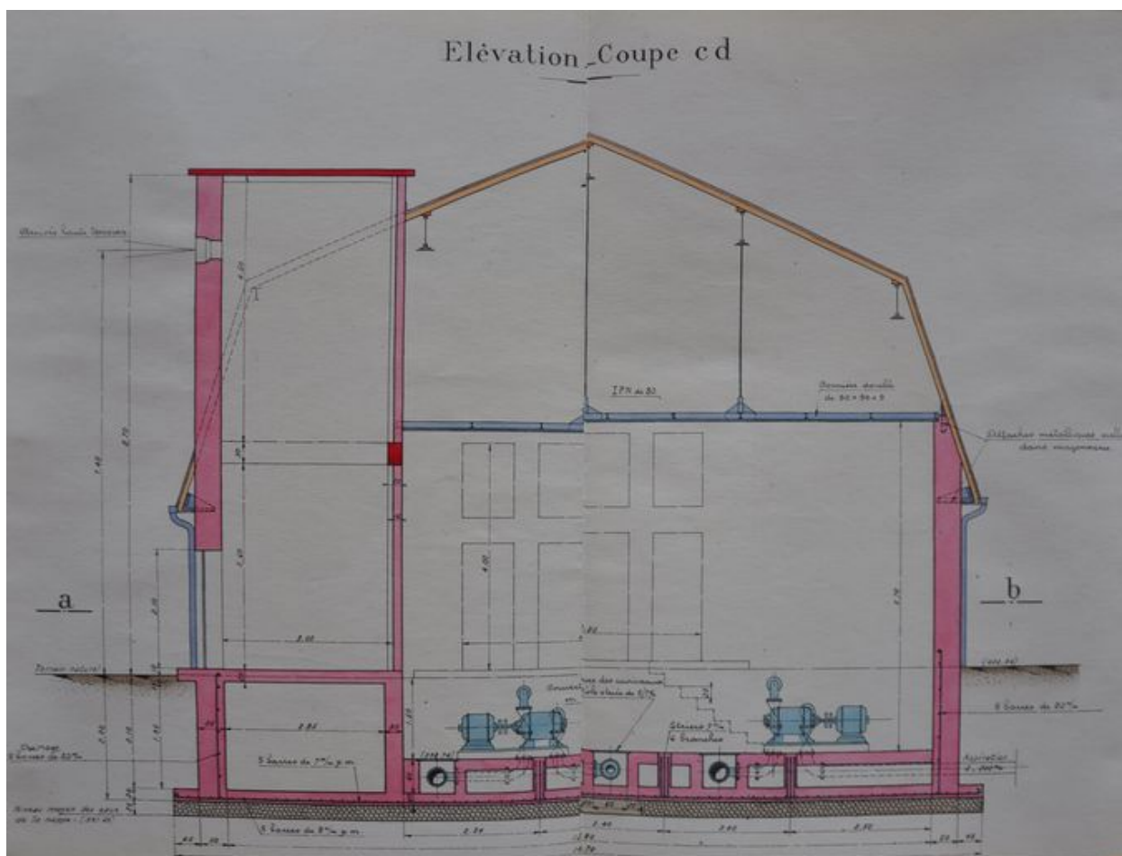
Station de pompage des Eaux-Belle, Plan-Coupe ab, 1939. Plan. Archives départementales de la Haute-Savoie © Archives départementales de la Haute-Savoie. 2 O 787/11
