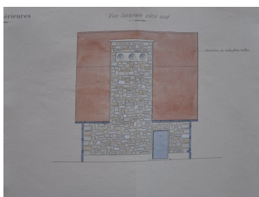
Station de pompage, plan, coupes, élévations : Profil-Coupe ef, 1939. Plan. Archives départementales de la Haute-Savoie © Archives départementales de la Haute-Savoie. 2 O 787/11 Phot. Samir Mahfoudi, Autr. Marc Merlin IVR82_20107400280NUCA
