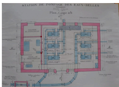
Plan d'ensemble, 1939. Plan. Archives départementales de la Haute-Savoie © Archives départementales de la Haute-Savoie. 2 O 787/10 Phot. Samir Mahfoudi, Autr. Ville d'Annemasse IVR82_20107400283NUCA
