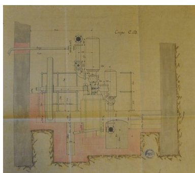
Coupe C.D. du bâtiment des pompes. Plan. Archives municipales d'Annemasse © Archives municipales d'Annemasse. 36/36 Phot. Samir Mahfoudi
