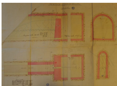
Réservoir des Eaux-Belles, Salève, 1923. Plan. Archives municipales d'Annemasse © Archives municipales d'Annemasse. 36/36 Phot. Samir Mahfoudi, Autr. Jean Visconti IVR82_20107400263NUCA
