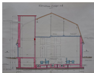
Station de pompage des Eaux-Belle, Plan-Coupe ab, 1939. Plan. Archives départementales de la Haute-Savoie © Archives départementales de la Haute-Savoie. 2 O 787/11 Phot. Samir Mahfoudi, Autr. Marc Merlin IVR82_20107400282NUCA
