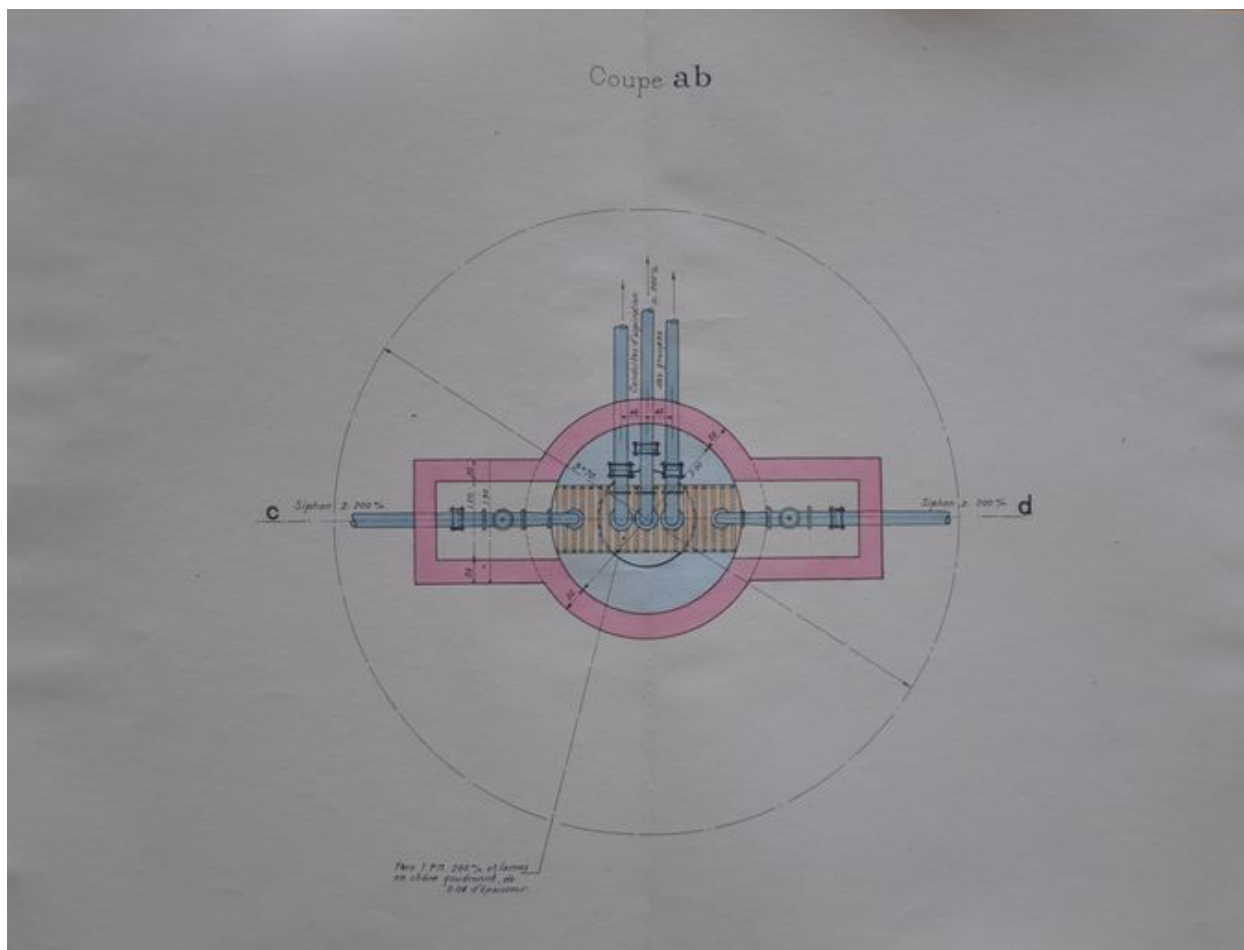
Station de pompage, plan, coupes, élévations : façade principale, 1939. Plan. Archives départementales de la Haute-Savoie © Archives départementales de la Haute-Savoie. 2 O 787/11
