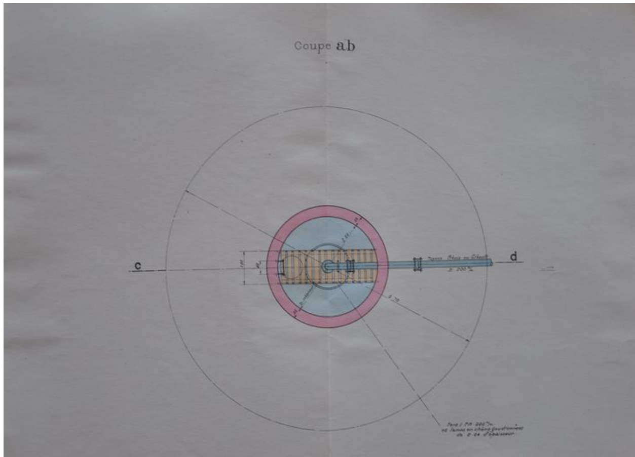
Puits de captage, coupes cd, 1939. Plan. Archives départementales de la Haute-Savoie © Archives départementales de la Haute-Savoie. 2 O 787/9
