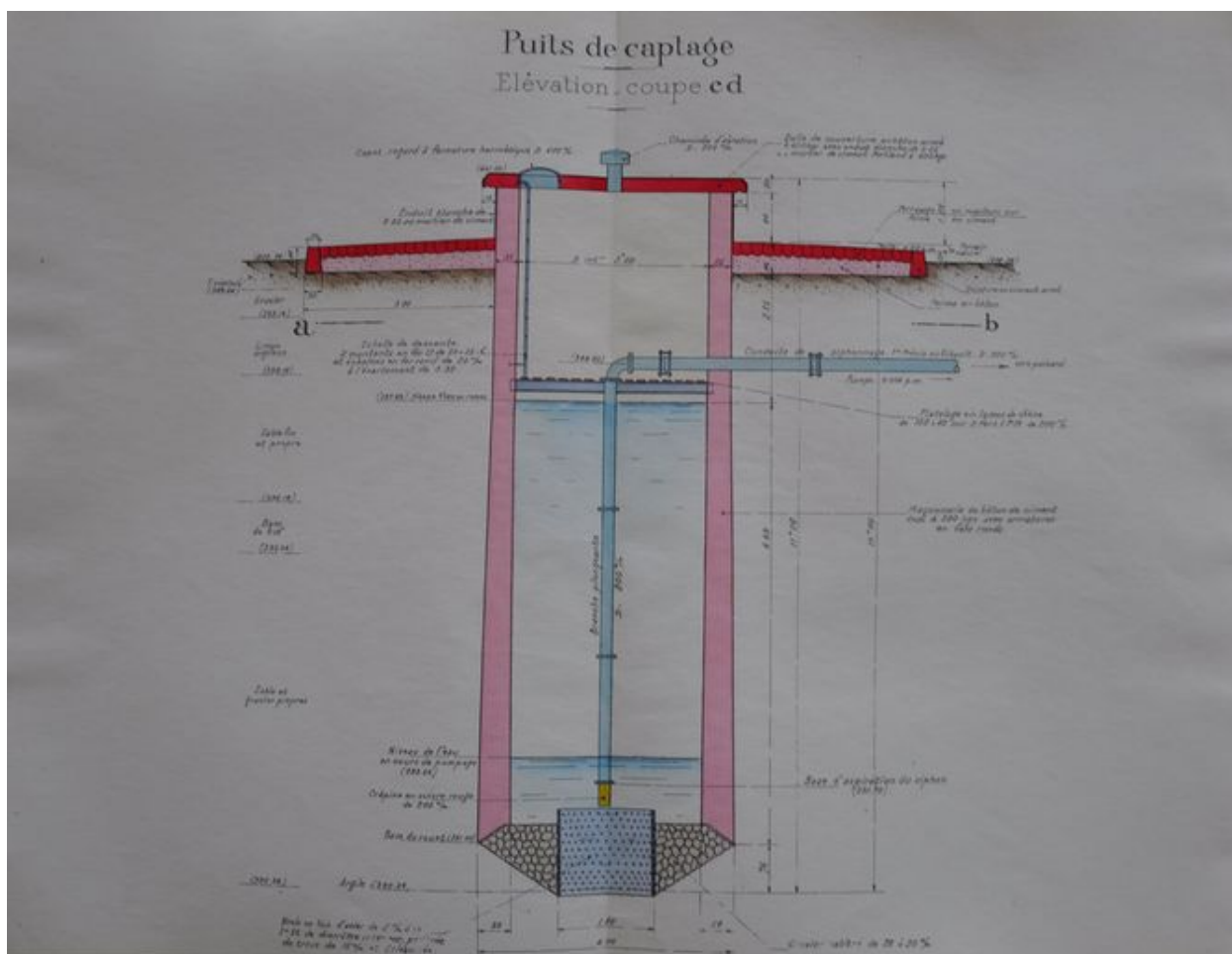
Puits de captage, coupes ab, 1939. Plan. Archives départementales de la Haute-Savoie © Archives départementales de la Haute-Savoie. 2 O 787/9
