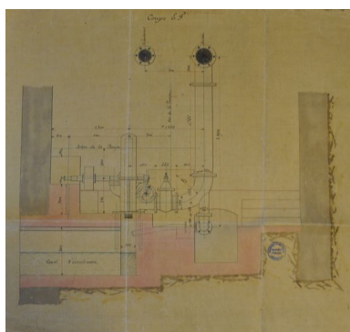
Coupe E.F. Plan. Archives municipales d'Annemasse © Archives municipales d'Annemasse. 36/36 Phot. Samir Mahfoudi IVR82_20107400266NUCA
