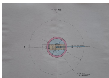
Puits de captage, coupes cd, 1939. Plan. Archives départementales de la Haute-Savoie © Archives départementales de la Haute-Savoie. 2 O 787/9 Phot. Samir Mahfoudi, Autr. Marc Merlin IVR82_20107400276NUCA
