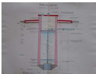
Puits de captage, coupes ab, 1939. Plan. Archives départementales de la Haute-Savoie © Archives départementales de la Haute-Savoie. 2 O 787/9 Phot. Samir Mahfoudi, Autr. Marc Merlin IVR82_20107400277NUCA
