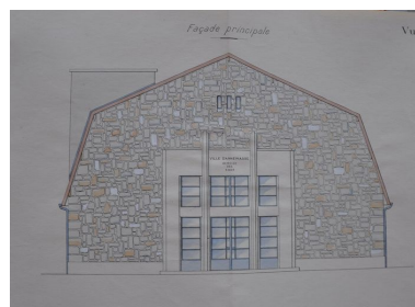
Station de pompage, plan, coupes, élévations : vue latérale côté sud, 1939. Plan. Archives départementales de la Haute-Savoie © Archives départementales de la Haute-Savoie. 2 O 787/11 Phot. Samir Mahfoudi, Autr. Marc Merlin IVR82_20107400279NUCA
