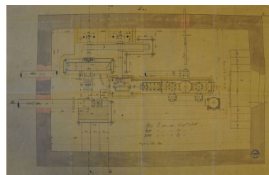
Pour M. Chavannes et Burnat, ingénieur domicilié à Lausanne, nouvelle pompe, 1883. Plan. Archives municipales d'Annemasse © Archives municipales d'Annemasse. 36/36 Phot. Samir Mahfoudi IVR82_20107400264NUCA
