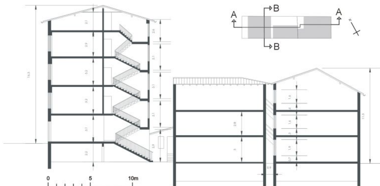
Coupe longitudinale
