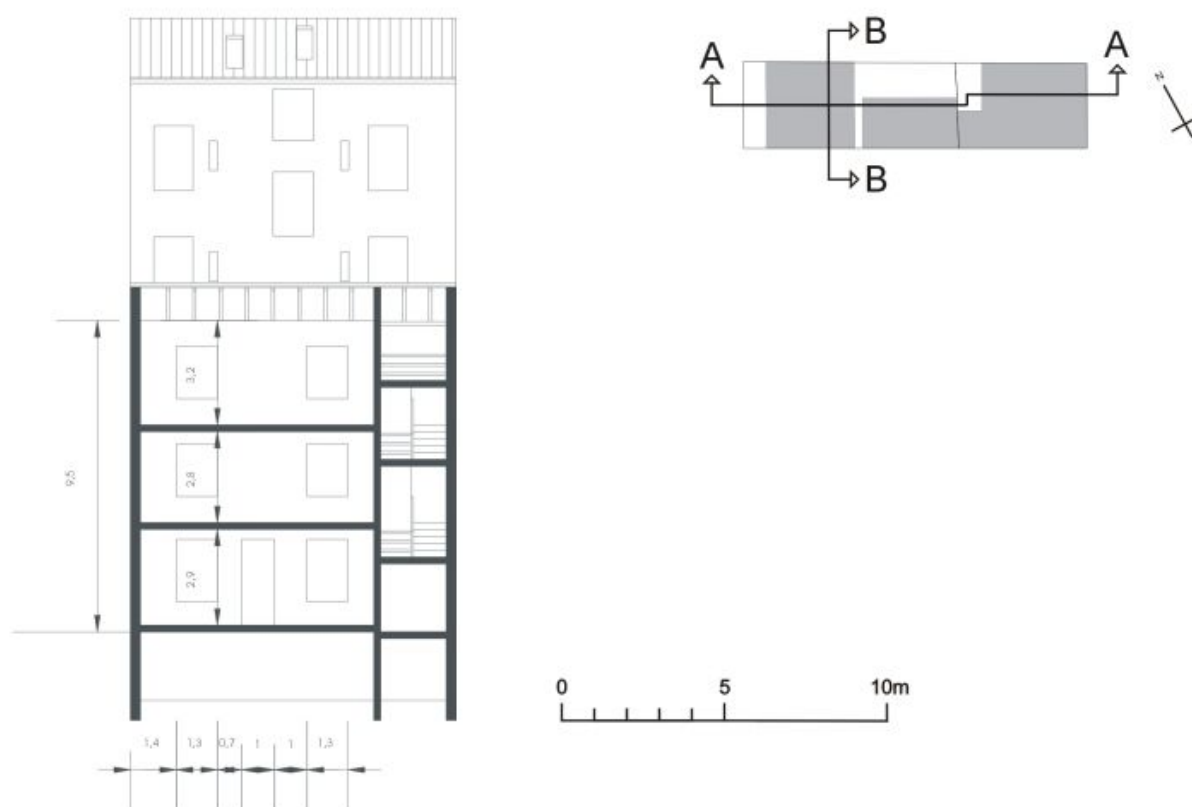
Coupe transversale
