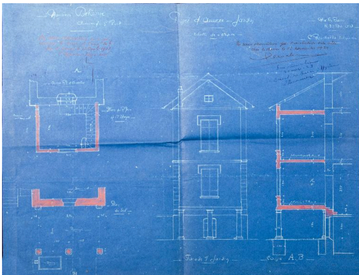
Agrandissement de 1923 : plan, coupe et élévation
