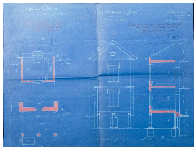
Agrandissement de 1923 : plan, coupe et élévation Repro. Denys Harreau IVR84_20177300236NUCB
