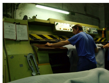
Vue d'ensemble de la tannerie : machines Phot. Nadine Halitim-Dubois IVR82_20102600699NUCA
