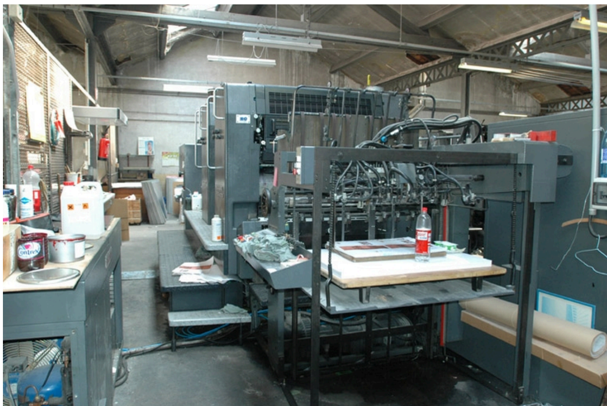
Machine offset quatre couleurs, vue avant (cf n°1 sur le plan).
