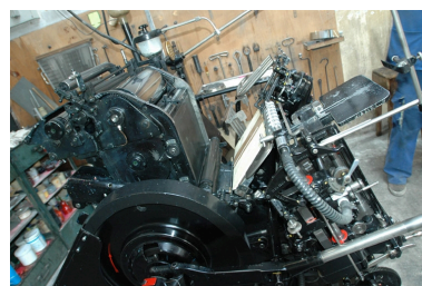
Heidelberg Platine (typo), vue sur la table d'impression. Phot. Nadine Halitim-Dubois IVR82_20096901783NUCA
