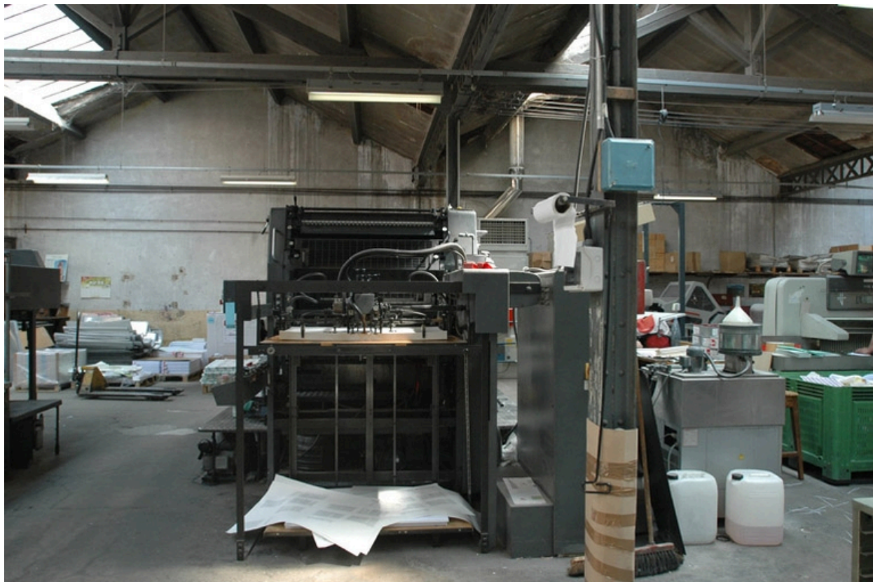
Machine offset quatre couleurs, vue avant (cf n°2 sur le plan).
