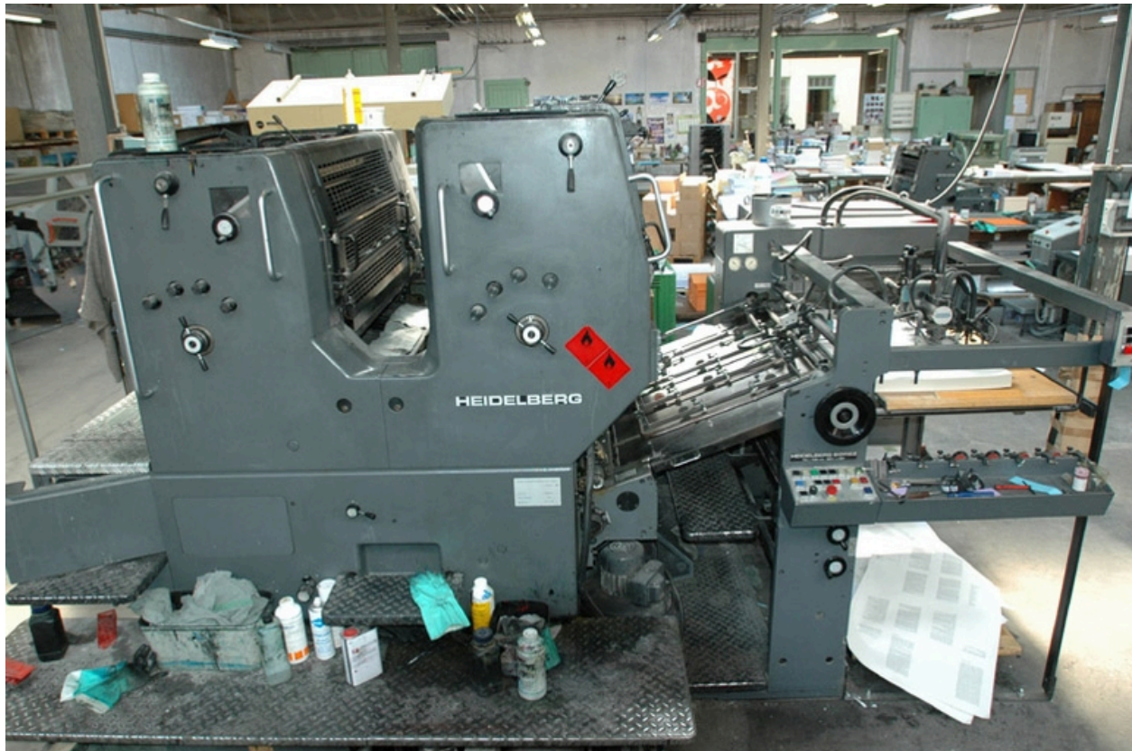
Machine offset quatre couleurs, partie latérale, (cf n°2 sur le plan).
