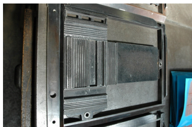
Châssis avec différents lingots et linotypes. Phot. Nadine Halitim-Dubois IVR82_20096901791NUCA
