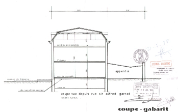
Coupe, 1988 Repro. François Fouger IVR82_20127300875NUCB
