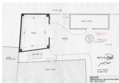
Remise : plan état initial, 1984 Repro. Denys Harreau IVR82_20137301112NUCB
