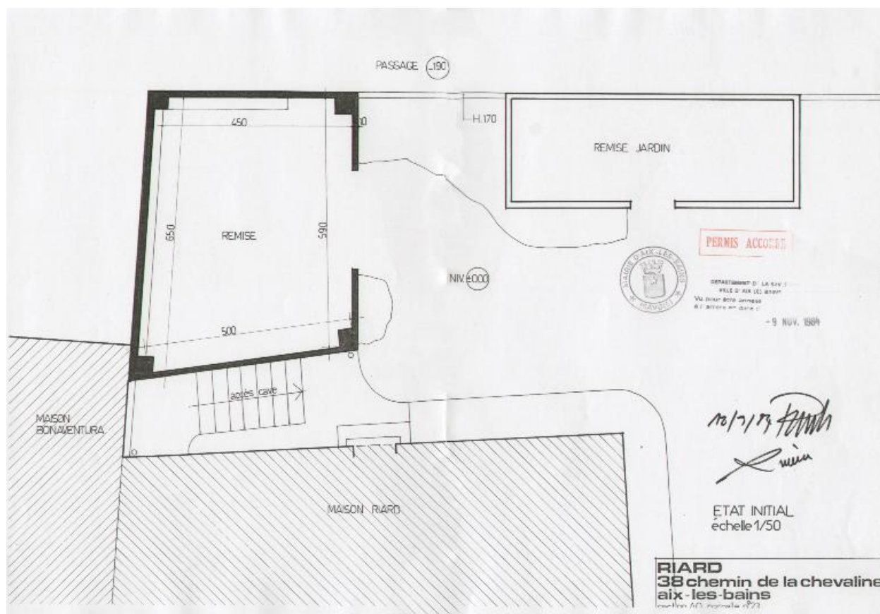
Remise : plan état initial, 1984
