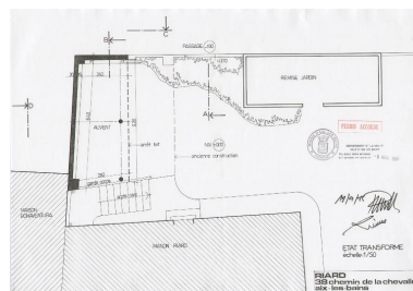
Remise : plan état transformé, 1984 Repro. Denys Harreau IVR82_20137301113NUCB
