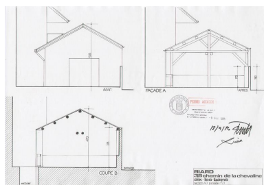
Remise : élévation, 1984 Repro. Denys Harreau IVR82_20137301114NUCB
