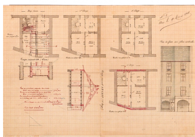
Plans, coupe et élévation Repro. François Fouger IVR82_20057300220NUCB
