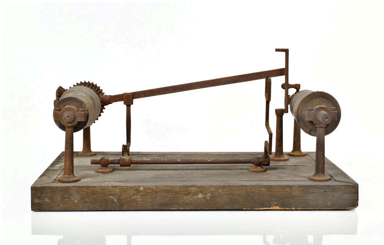
Variateur de vitesse, vue 1
