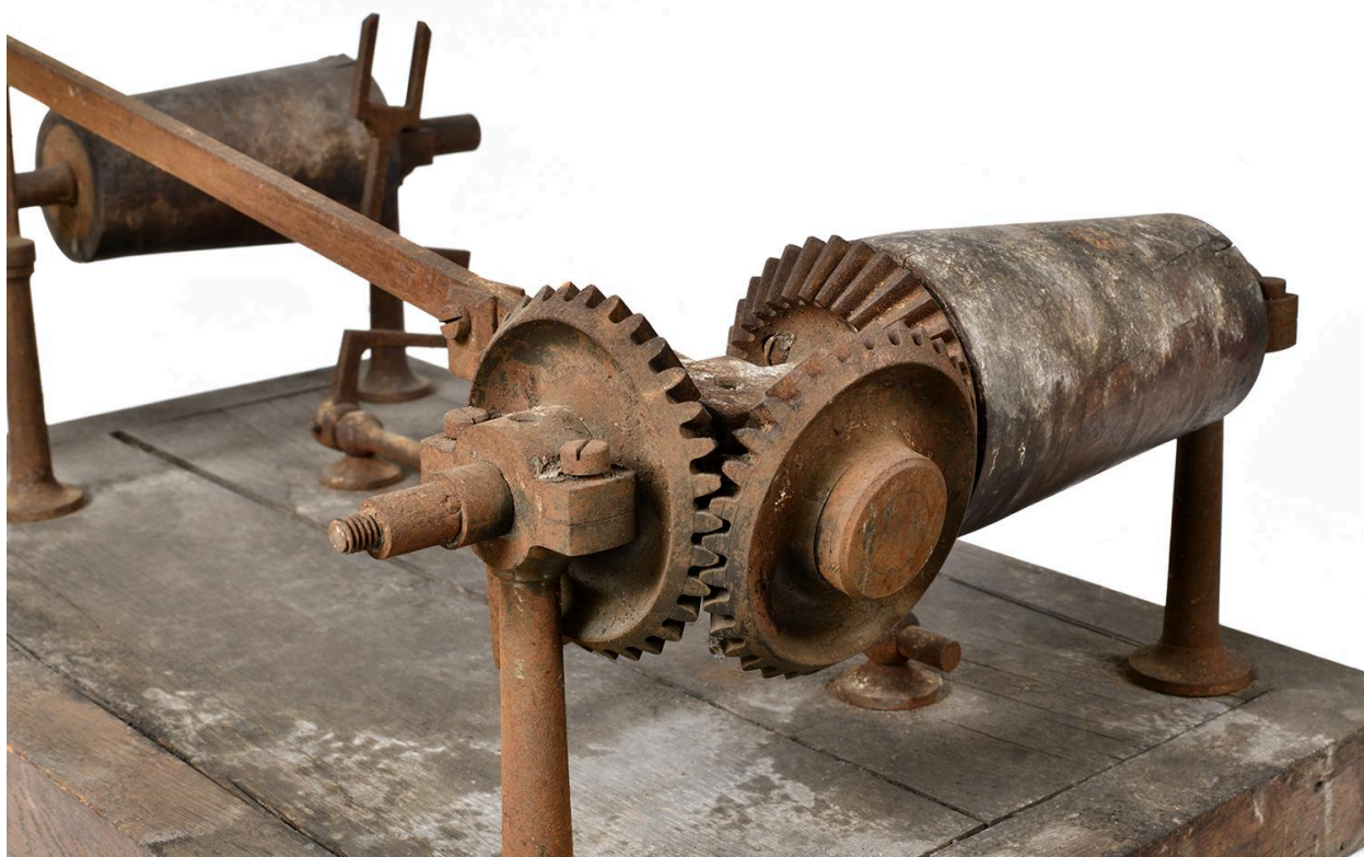
Variateur de vitesse, vue 3, vue de détail
