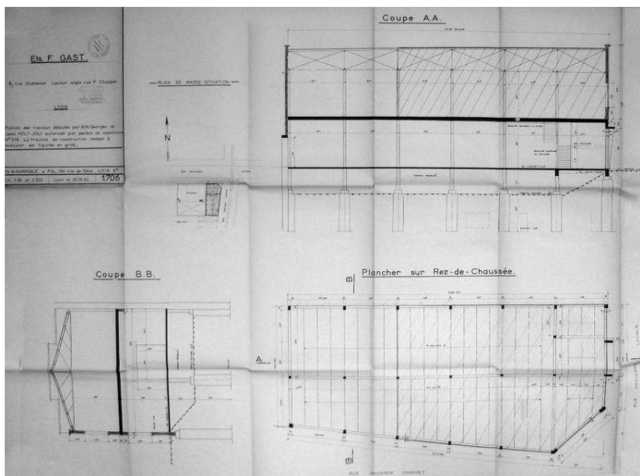
Plans et coupes, Ets GAST, 6 rue Challemeil Lacour, 1962. (Arch. mun. Lyon)
