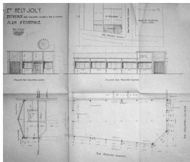
Plans d'ensemble, Ets HELY JOLY Entrepôt, 6 rue Challemel Lacour, 28 mai 1956 par Yvon Meunier architecte, échelle 1/100. (Arch. mun. Lyon) Phot. Salohy Rakotomalala IVR82_20106901486NUC
