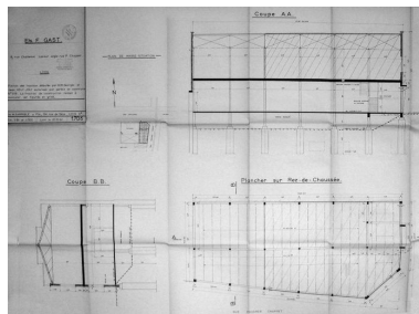
Plans et coupes, Ets GAST, 6 rue Challemel Lacour, 1962. (Arch. mun. Lyon) Phot. Salohy Rakotomalala IVR82_20106901487NUC
