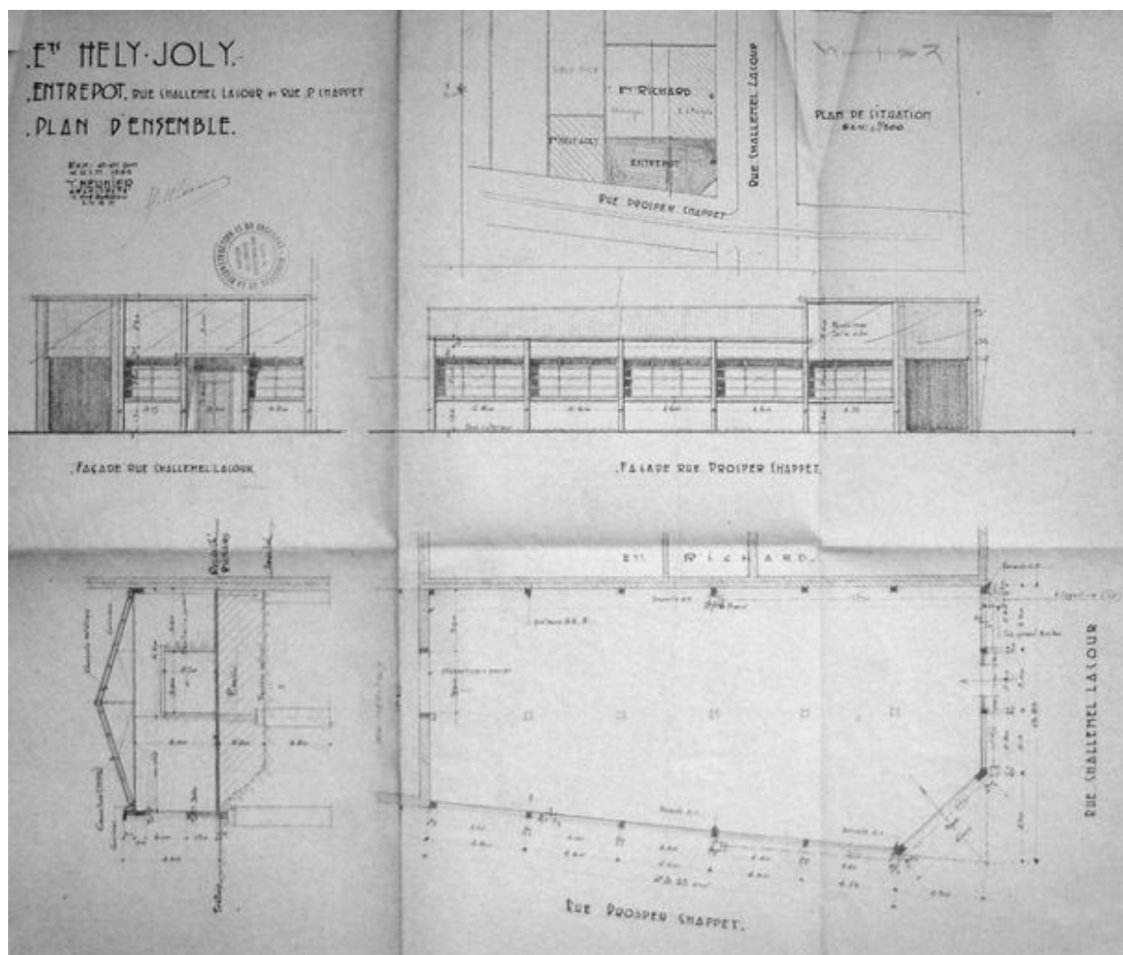
Plans d'ensemble, Ets HELY JOLY Entrepôt, 6 rue Challeml Lacour, 28 mai 1956 par Yvon Meunier architecte, échelle 1/100. (Arch. mun. Lyon)
