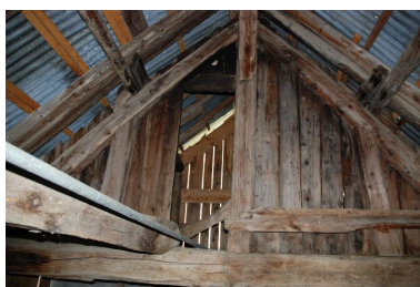
Vue de la charpente de l'étable. Phot. Thierry Monnet IVR84_20167306725NUCA
