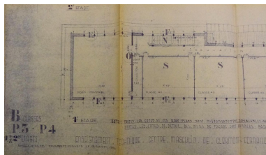
Bâtiment B (externat). Plans 1er (et 2e étage), partie gauche, par A. Aubert, et A. Blanc, 15 janvier 1954. Phot. Bénédicte Renaud-Morand IVR84_20236300235NUCA
