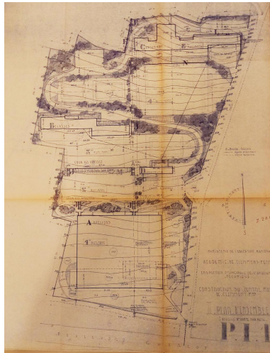
Plan d'ensemble, [1956 ] (AC Clermont-Ferrand, permis de construire n°2261) Repro. Bénédicte Renaud-Morand IVR84_20236300225NUCA
