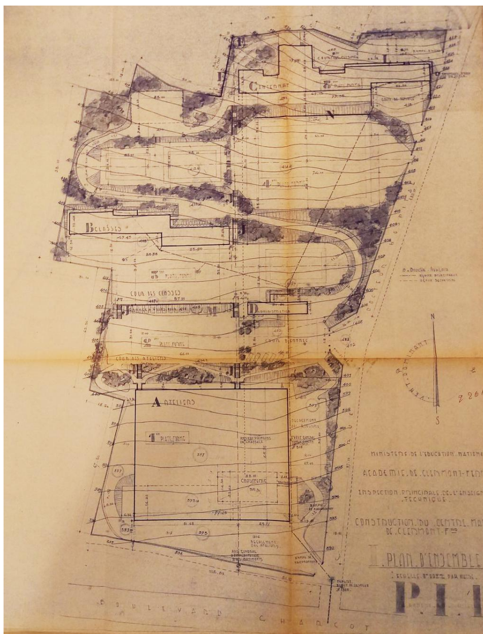
Plan d'ensemble, [1956] (AC Clermont-Ferrand, permis de construire n°2261)
