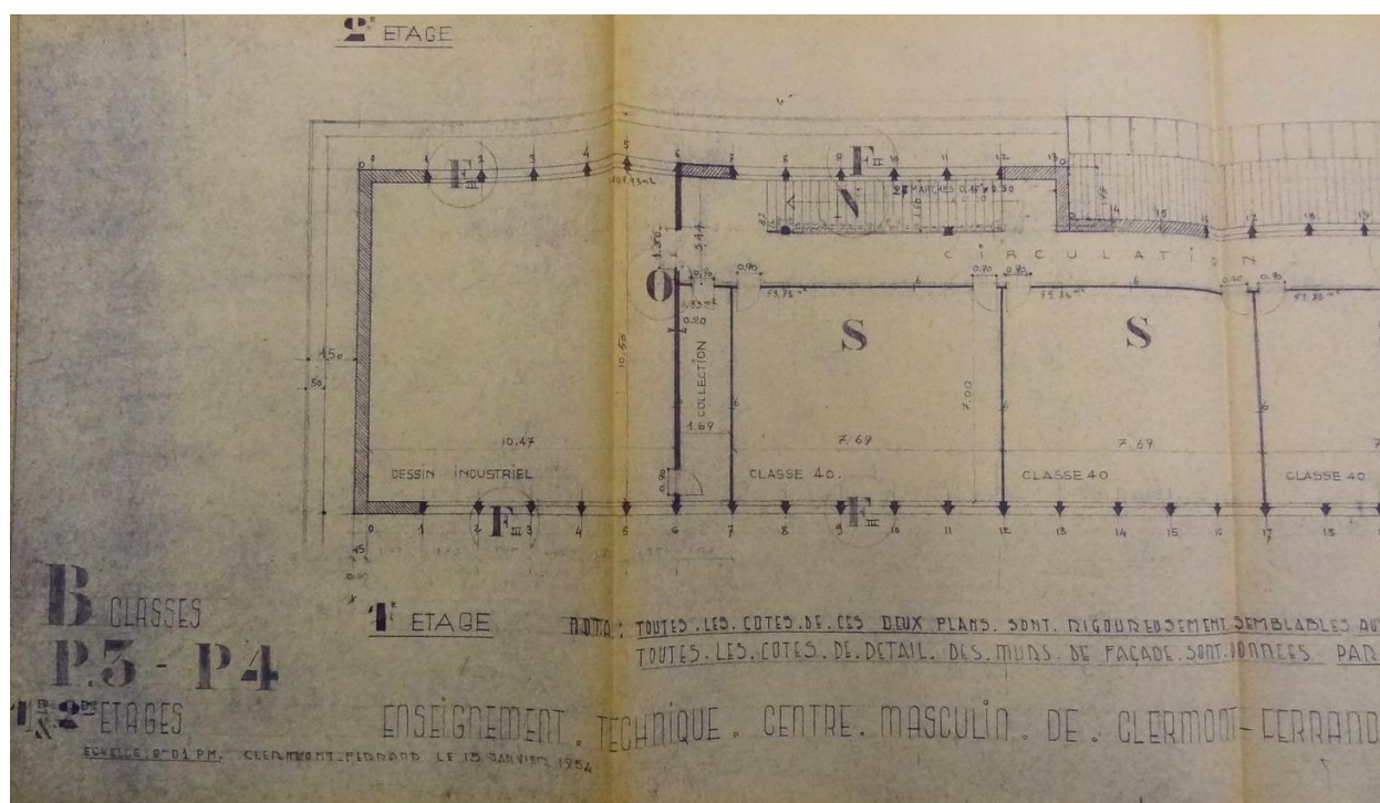
Bâtiment B (externat). Plans 1er (et 2e étage), partie gauche, par A. Aubert, et A. Blanc, 15 janvier 1954.
