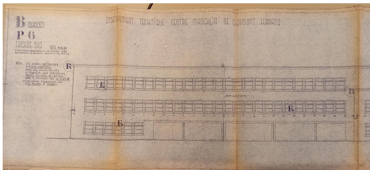
Bâtiment B (externat : les classes). Façade sud, par A. Aubert et A. Blanc, 15 janvier 1954.
