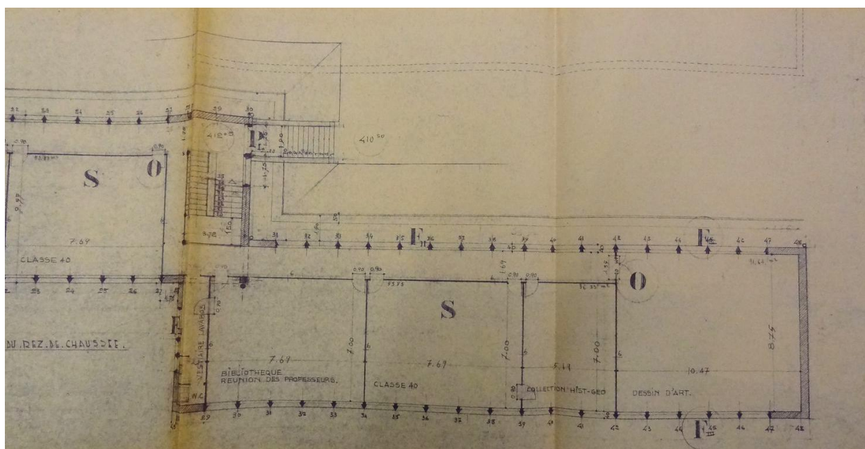
Bâtiment B (externat). Plans 1er (et 2e étage), partie droite, par A. Aubert, et A. Blanc, 15 janvier 1954.
