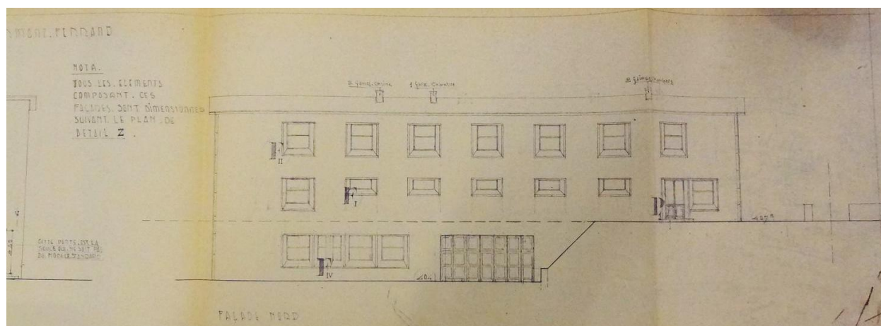
Bâtiment D (administration). Façade nord, [par A. Aubert et A. Blanc], 15 janvier 1954.
