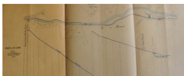
Projet de construction d'une centrale électrique faisant apparaître le moulin, 1914 (FR.AD073, 82S31). IVR84_20167302577NUCA
