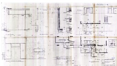
Détails de la liaison avec l'immeuble Cassiopée. Marcel Breuer architecte, 18 juin 1971. Modifié les 1er et 13 juillet 1971 (AC Arâches-la Frasse) Phot. Jean-François Lyon-Caen, Phot. C. Salomon-Pelen IVR82_20127401284NUC
