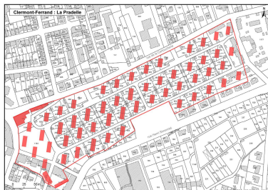
Plan des différents bâtiments d'origine de la cité. Dess. Guylaine Beauparland-Dupuy IVR84_20216301266NUDA
