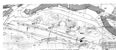
Plan masse. Plan de situation / J. Labro, A. Wujek, 17 novembre 1982 (AC Morzine) Phot. Jean-François Lyon- Caen, Phot. C. Salomon-Pelen IVR82_20087400421NUC
