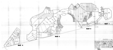
Plan de toiture / J. Labro, A. Wujek, 17 novembre 1982 (AC Morzine) Phot. Jean-François Lyon- Caen, Phot. C. Salomon-Pelen IVR82_20087400425NUC
