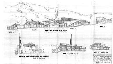
Coupe sur la place centrale, élévation nord sur rue, élévation ouest du bâtiment 3, élévation est du bâtiment 4 / J. Labro, A. Wujek, 17 novembre 1982 (AC Morzine) Phot. Jean-François Lyon- Caen, Phot. C. Salomon-Pelen IVR82_20087400427NUC
