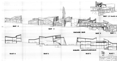
Coupe longitudinale, élévation sud, élévation est des bâtiments 1 et 2 / J. Labro, A. Wujek, 17 novembre 1982 (AC Morzine) Phot. Jean-François Lyon- Caen, Phot. C. Salomon-Pelen IVR82_20087400426NUC
