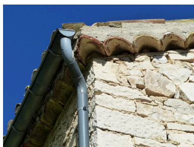
Angle sud-ouest, passage du rang de génoise de l'avant-toit vers la saillie de rive.
