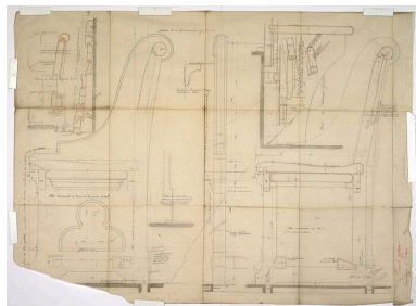
Dessins d'exécution des bancs (AP Eglise Réformée de Lyon, Gaspard André). Repro. Didier Gourbin, Autr. Gaspard André IVR82_20106906116NUCA
