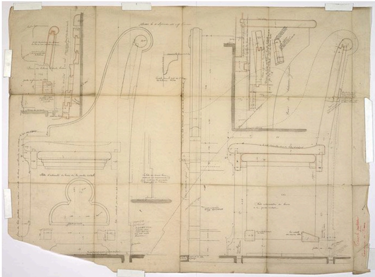
Dessins d'exécution des bancs (AP Eglise Réformée de Lyon, Gaspard André).
