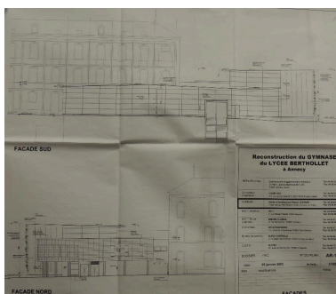
Élévation façades sud et nord Repro. Pascal Lemaître, Autr. Pascal Legrand IVR82_20147401578NUCA
