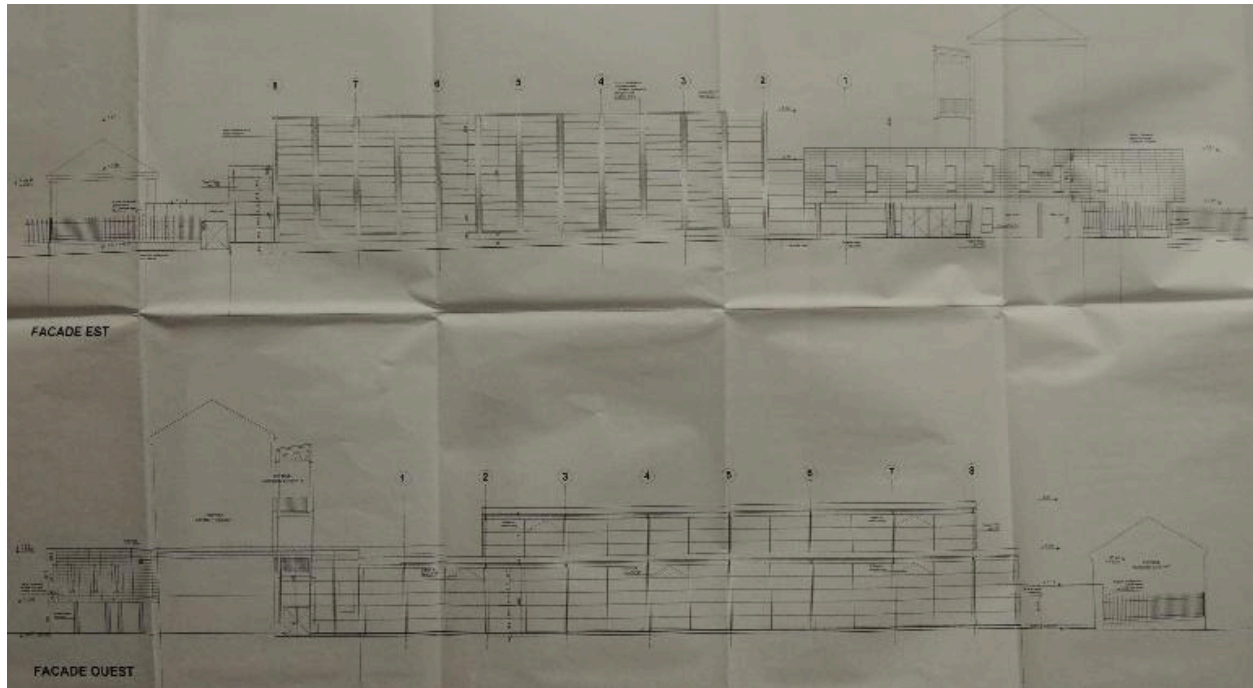
Élévation façades est et ouest
