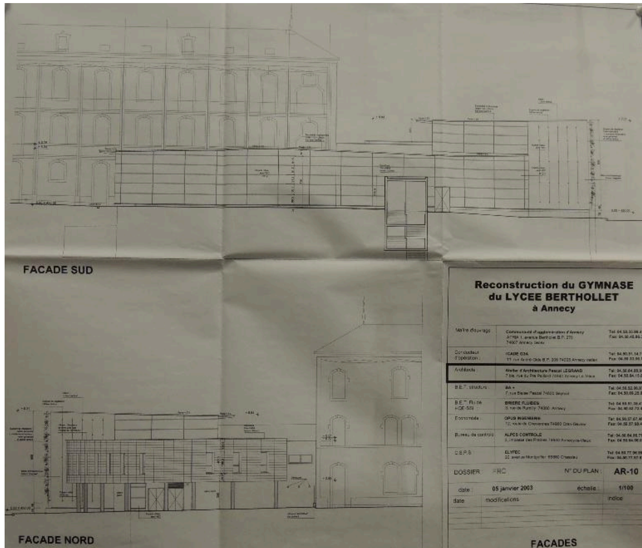
Élévation façades sud et nord
