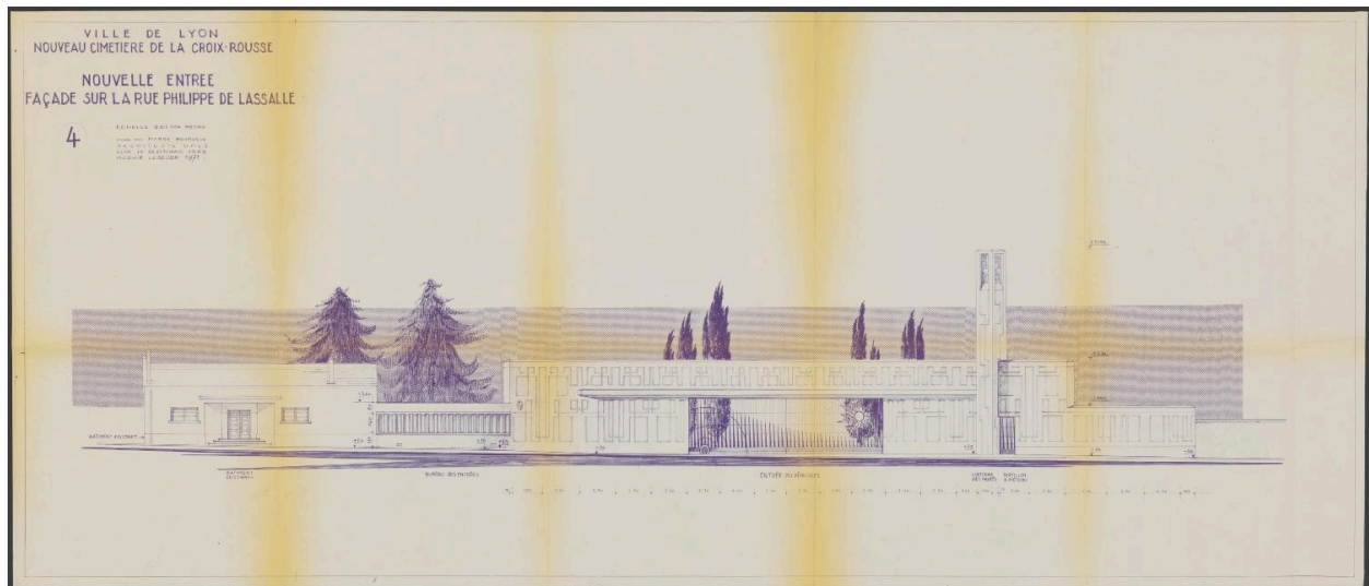
Elévation de la nouvelle entrée rue Philippe-de-Lassalle, 4, 1969, modifié en 1971
