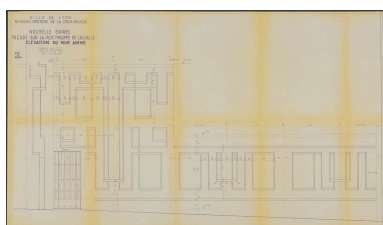
Elévation du mur animé, partie située au nord de la lanterne des morts, 21 avril 1970 Repro. Gilles Bernasconi IVR84_20256901640NUCA
