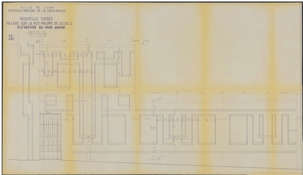
Elévation du mur animé, partie située au nord de la lanterne des morts, 21 avril 1970
