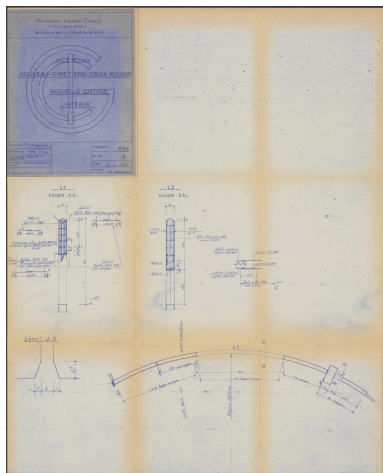
Plans et coupes des linteaux, Groupement Ingénieurs Conseils, 1972 Repro. Gilles Bernasconi IVR84_20256901626NUCA
