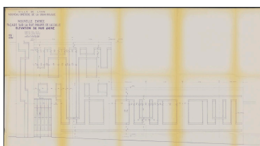
Elévation du mur animé, partie située au nord de la lanterne des morts, 21 avril 1970, modifié le 30 juin 1971 Repro. Gilles Bernasconi IVR84_20256901641NUCA
