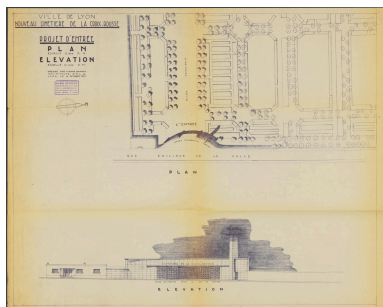
Plan et élévation sur la rue Philippe-de-Lassalle, 12 octobre 1955 Repro. Gilles Bernasconi IVR84_20256901862NUCA
