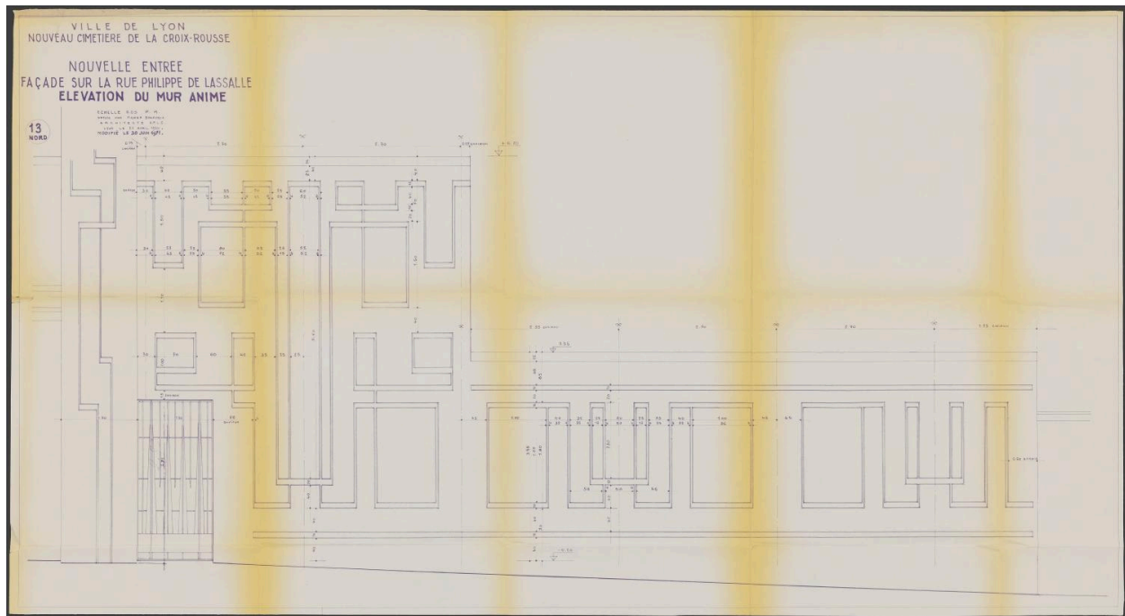
Elévation du mur animé, partie située au nord de la lanterne des morts, 21 avril 1970, modifié le 30 juin 1971
