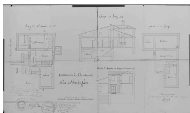
Plan et coupe de l'ancien presbytère (A3 493), devenu aujourd'hui résidence secondaire. Phot. Alain Franchella IVR82_19972600530X
