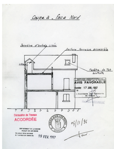
Coupe transversale Repro. François Fouger IVR82_20117300727NUCB
