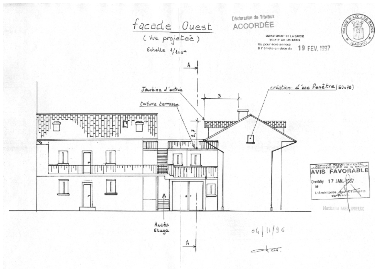
Elévation ouest
