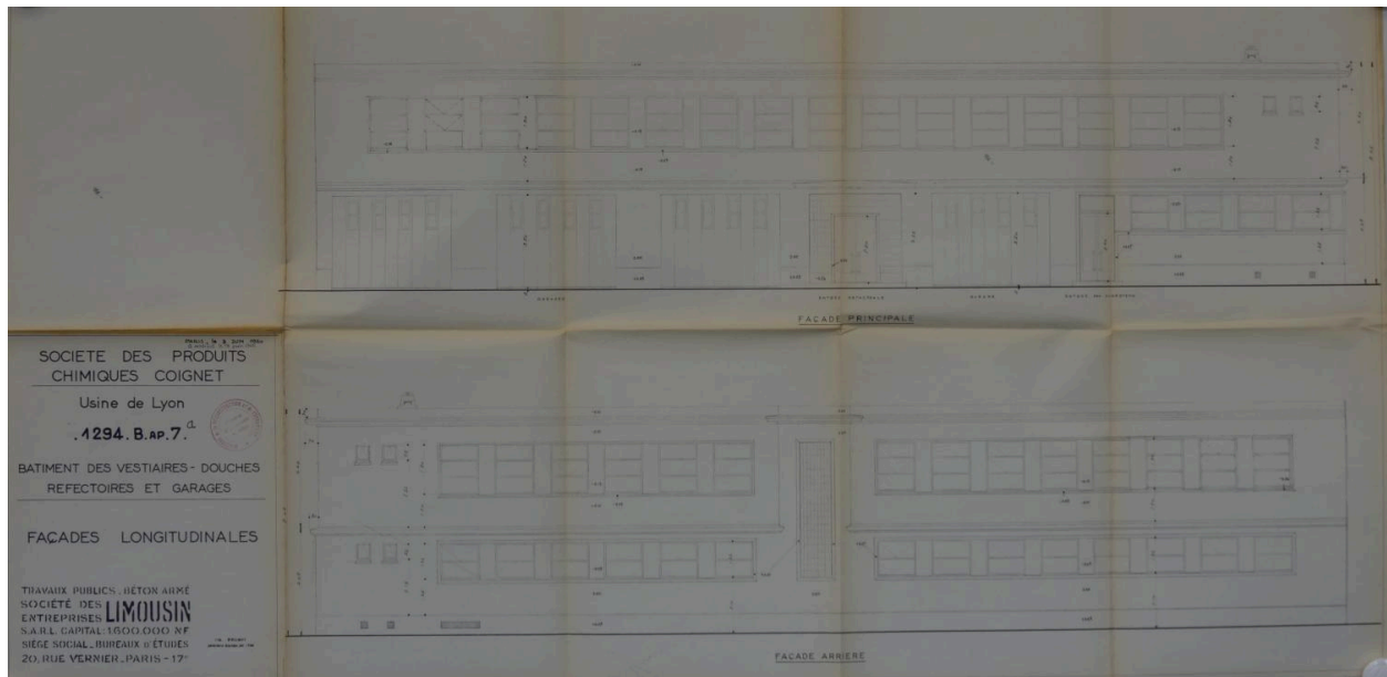
Façades longitudinales usine chimique Coignet 1960 (ACL 314W 296)
