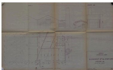
Plan détail alignement bld des Etats-Unis de l'usine chimique Coignet 1960 (ACL 314W 296) Phot. Nadine Halitim-Dubois IVR84_20256901427NUCA
