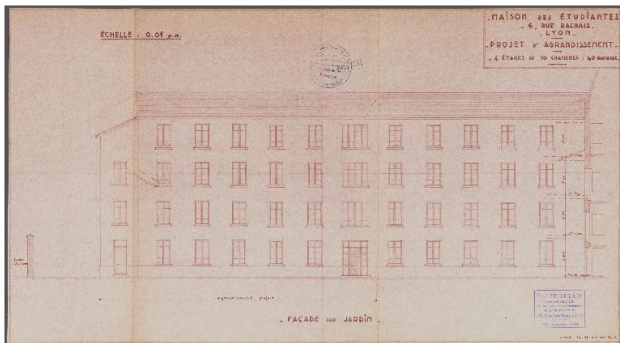
Projet d'élévation sur le jardin de l'aile des chambres, dans le cadre de son doublement, en 1950 (Arch. mun. Lyon, Paul Bellemain, tirage d'architecte, 345 W 24, n°433).
