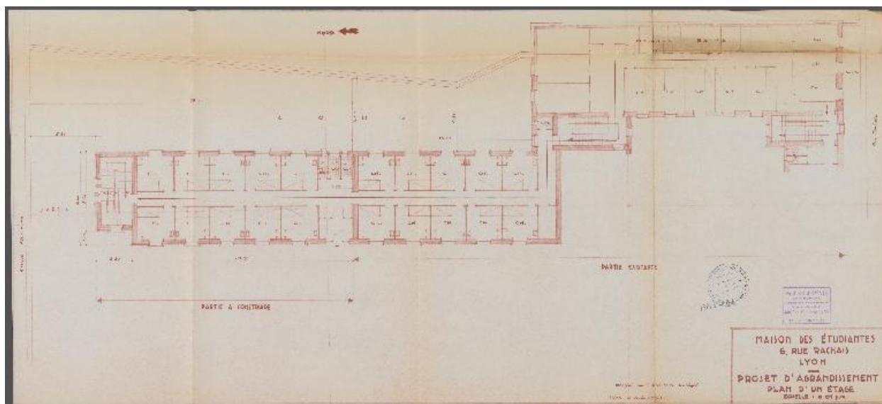
Plan type d'un étage, dans le cadre du projet de doublement de l'aile des chambres du foyer d'étudiantes, en 1950 (Arch. mun. Lyon, Paul Bellemain, tirage d'architecte, 345 W 24, n°433).
