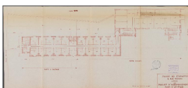
Plan type d'un étage, dans le cadre du projet de doublement de l'aile des chambres du foyer d'étudiantes, en 1950 (Arch. mun. Lyon, Paul Bellemain, tirage d'architecte, 345 W 24, n°433).
