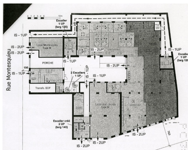
Plan masse du site, archives DAU ville de Lyon Phot. Nadine Halitim-Dubois IVR82_20086901879NUC
