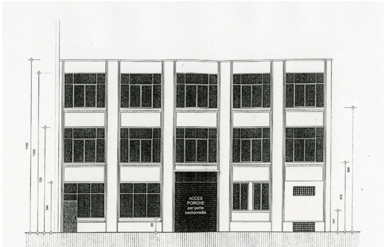
Façade nord (rue Montesquieu) DAU ville de Lyon
