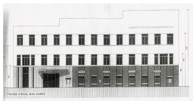
Façade principale (ouest) (archives DAU ville de Lyon) Phot. Nadine Halitim-Dubois IVR82_20086901878NUC
