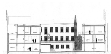
Coupe, cheminée, archives DAU ville de Lyon Phot. Nadine Halitim-Dubois IVR82_20086901880NUC
