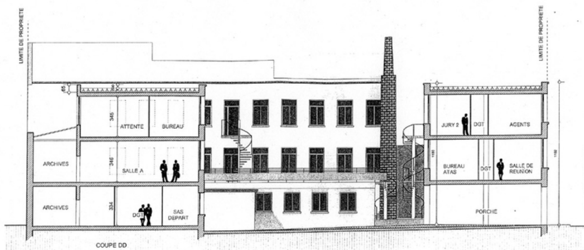
Coupe, cheminée, archives DAU ville de Lyon
