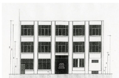
Façade nord (rue Montesquieu) DAU ville de Lyon Phot. Nadine Halitim-Dubois IVR82_20086901881NUC
