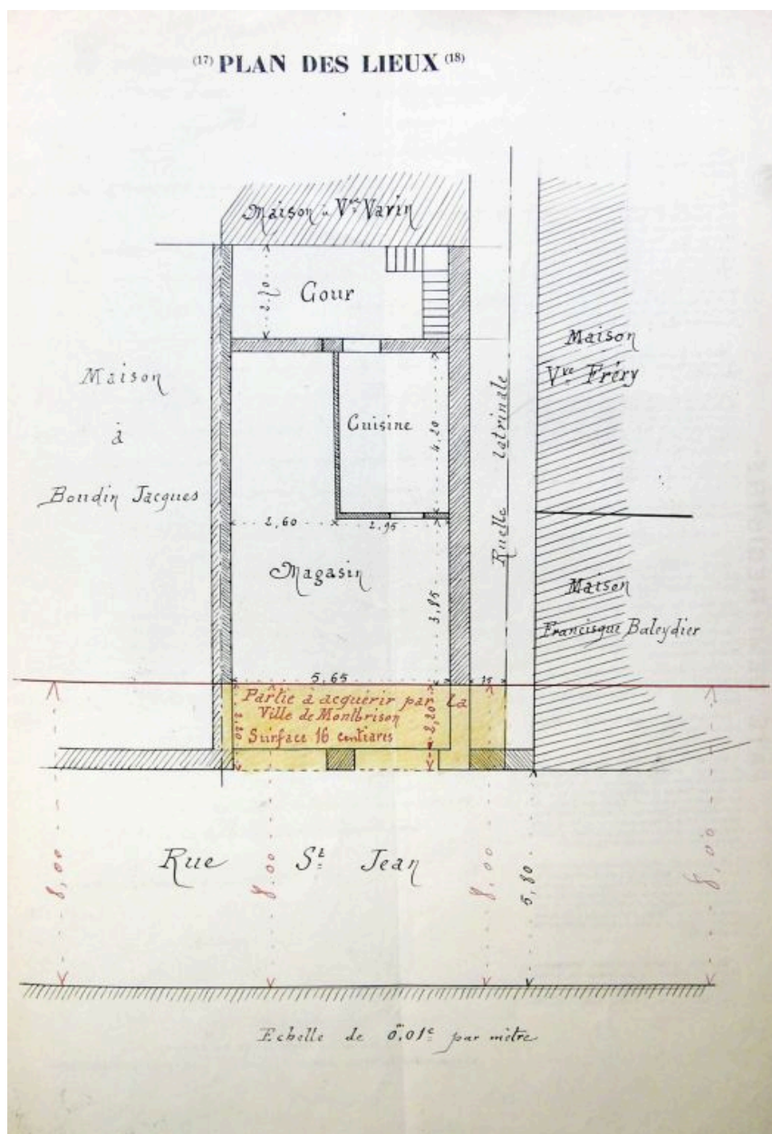
Plan des lieux, 4 rue Saint-Jean.
