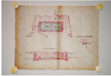
AC Pugny-Chatenod. Archives : Sources. Plans du bassin double, coupe longitudinale, coupe de la chambrette. [vers 1895] Phot. Thierry Monnet IVR84_20177300742NUCA
