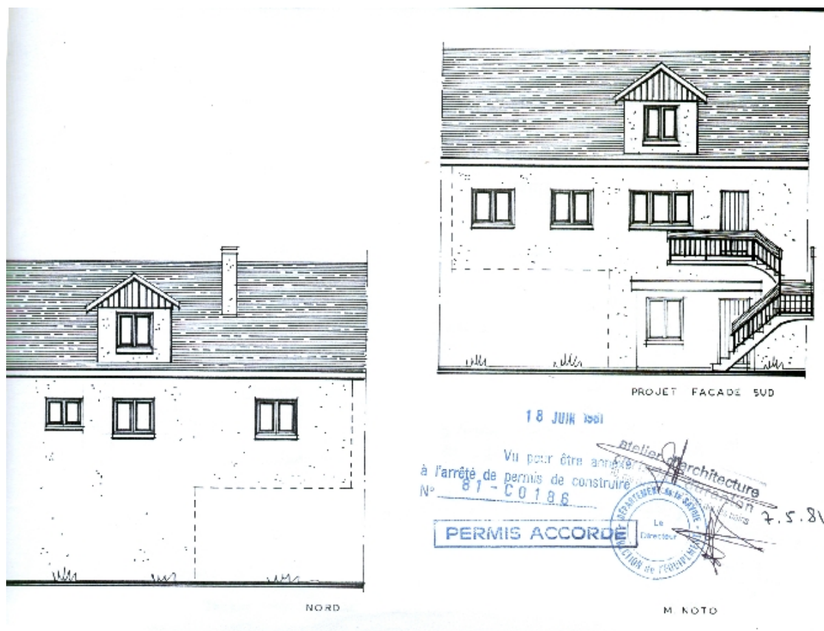
Elévations nord et sud
