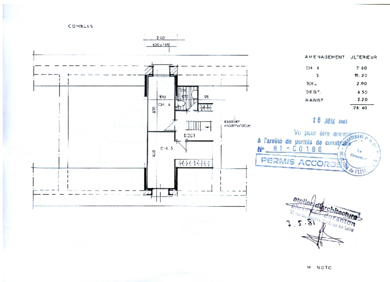
Plan des combles
