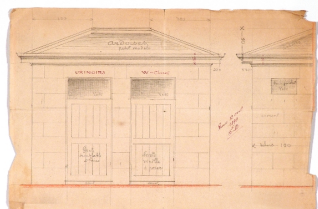
Elévation des vespasiennes Repro. François Fouger IVR82_20057300070NUCB
