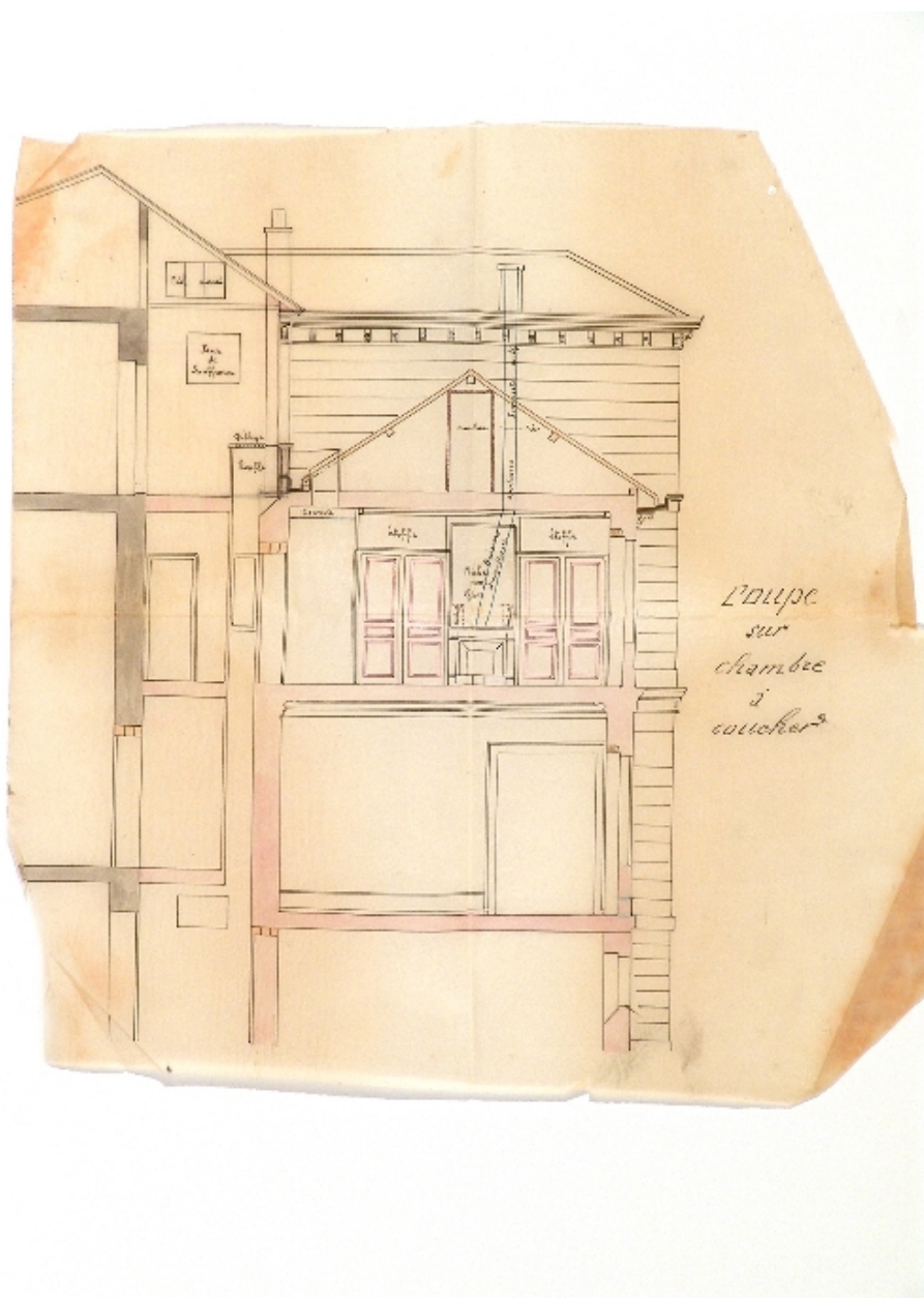
Maison Numa Blanc : coupe sur la chambre à coucher
