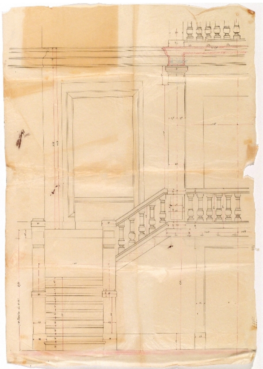
Maison Numa Blanc : élévation de l'escalier
