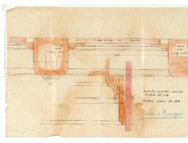
Maison Numa Blanc : détail de moulures de la salle à manger Repro. François Fouger IVR82_20057300072NUCB
