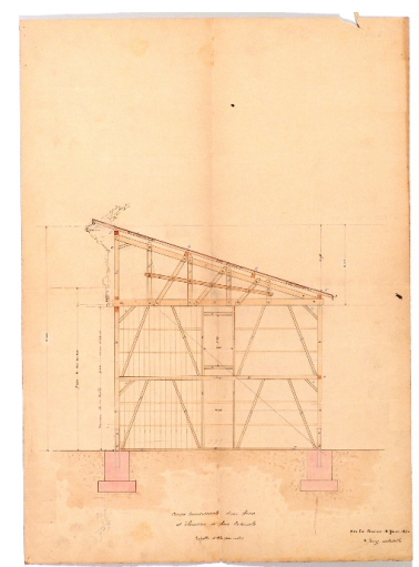
Atelier de photographies : coupe transversale d'une ferme Repro. François Fouger IVR82_20057300071NUCB
