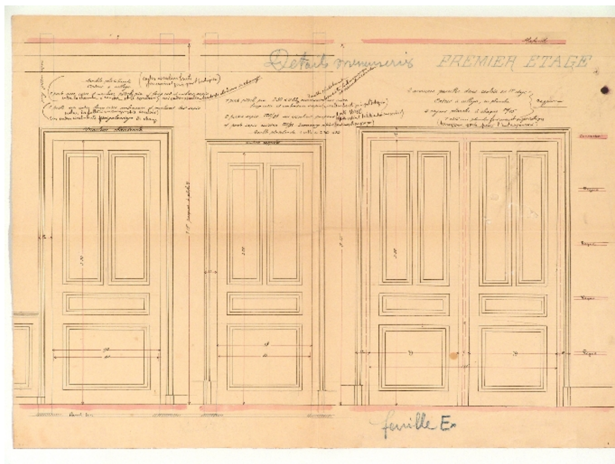
Maison Numa Blanc : détail de menuiserie au 1er étage
