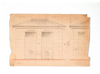
Elévation des vespasiennes Repro. François Fouger IVR82_20057300070NUCB
