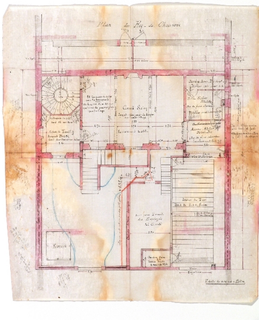
Maison Numa Blanc : plan du rez-de-chaussée
