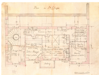
Maison Numa Blanc : plan du 1er étage Repro. François Fouger IVR82_20057300066NUCB
