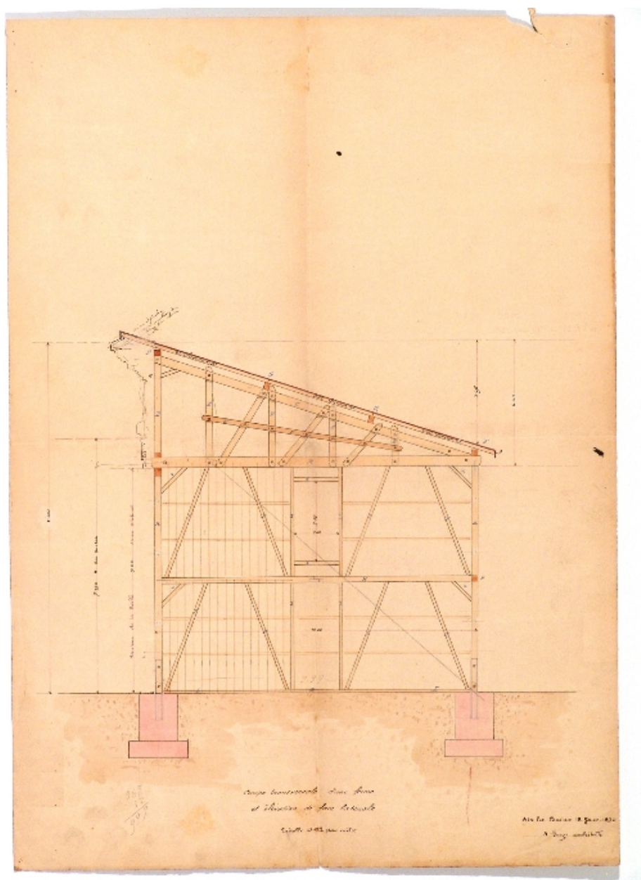
Atelier de photographies : coupe transversale d'une ferme
