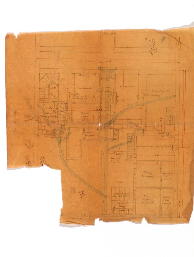
Maison Numa Blanc : plan du sous-sol Repro. François Fouger IVR82_20057300064NUCB
