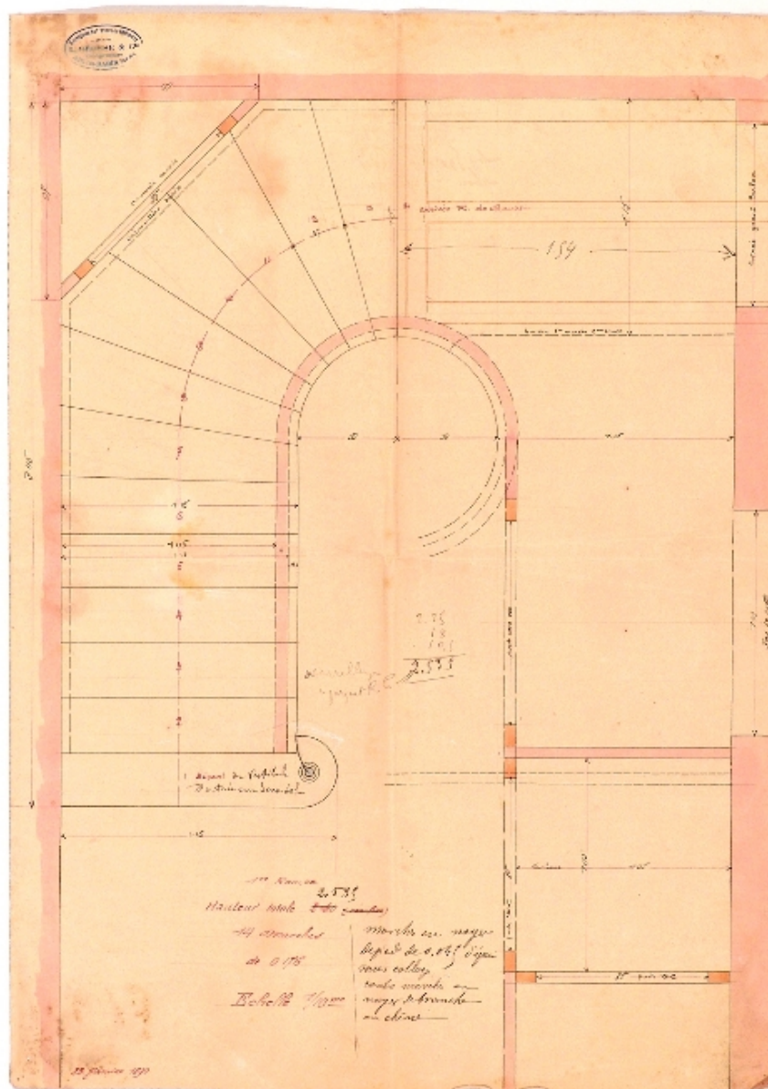
Maison Numa Blanc : plan de l'escalier
