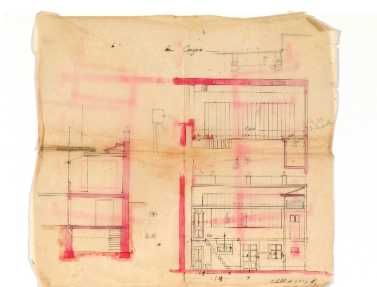
Atelier de photographies : coupe Repro. François Fouger IVR82_20057300069NUCB
